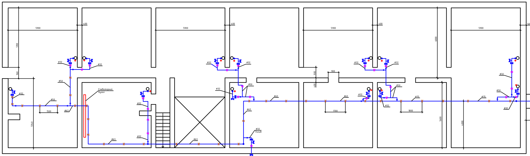
План підвалу першого під'їзду зі схемою прокладання трубопроводів системи водопостачання холодної води ( В1 )
