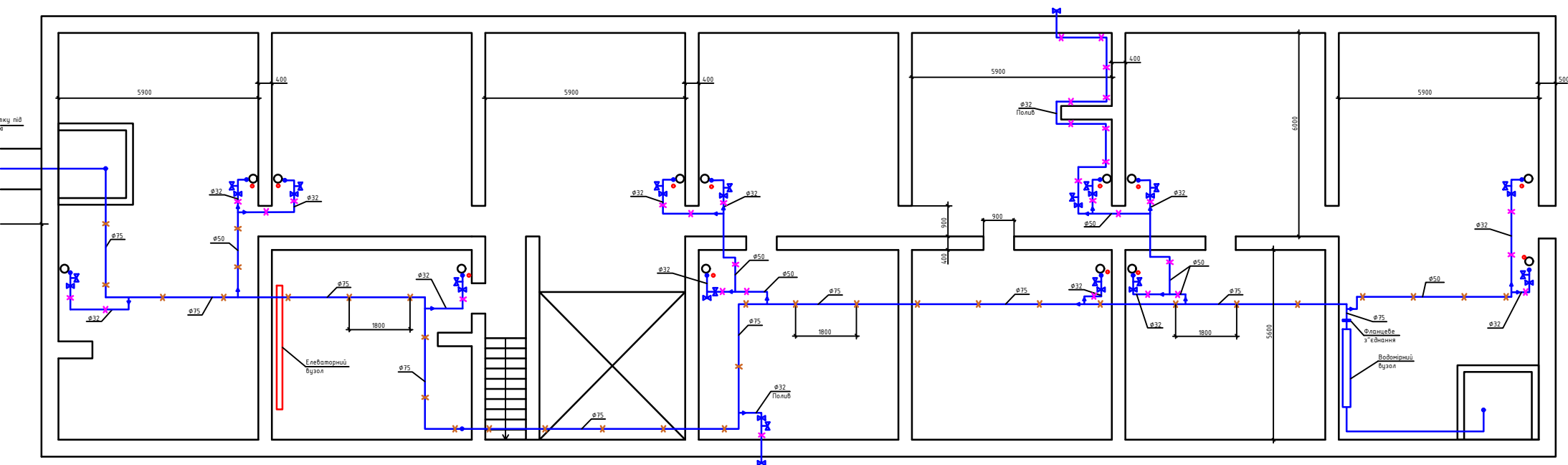
План підвалу другого під'їзду зі схемою прокладання трубопроводів системи водопостачання холодної води ( В1 )
