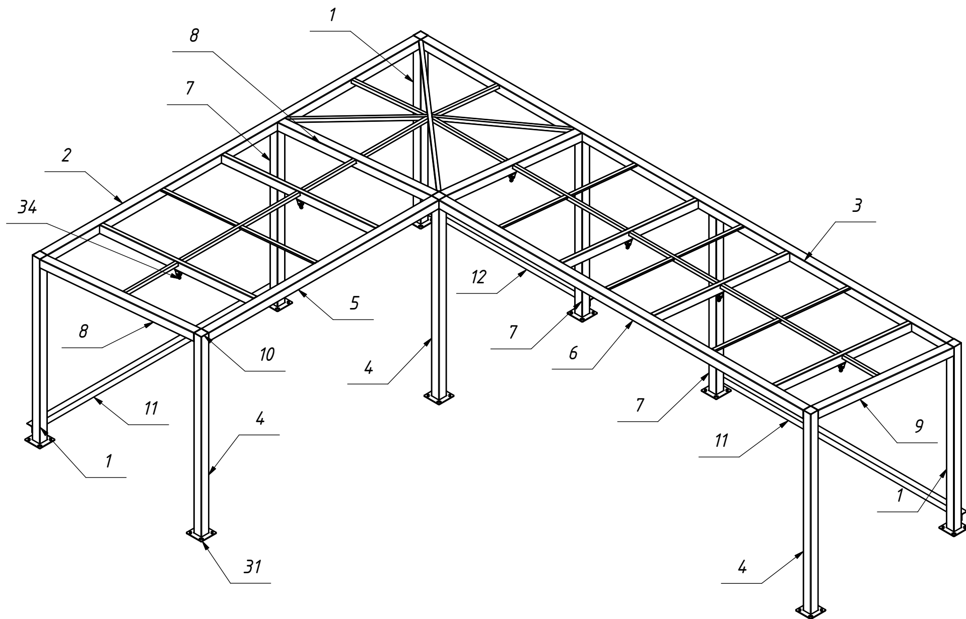
Какас перголи ( 1 : 25 )
