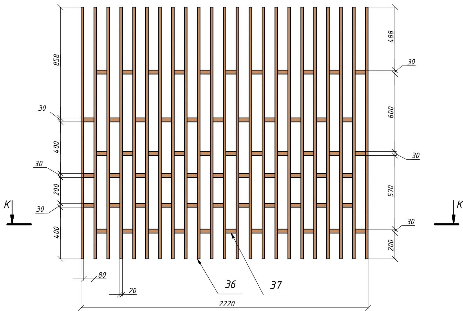
Ламелі (Модуль №2) ( 1 : 12 )
