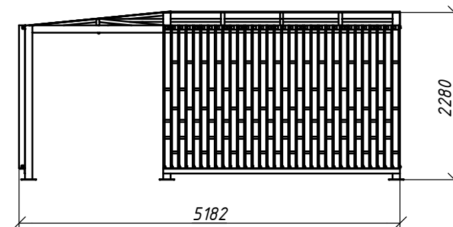
Вид збоку ( 1 : 50 )
