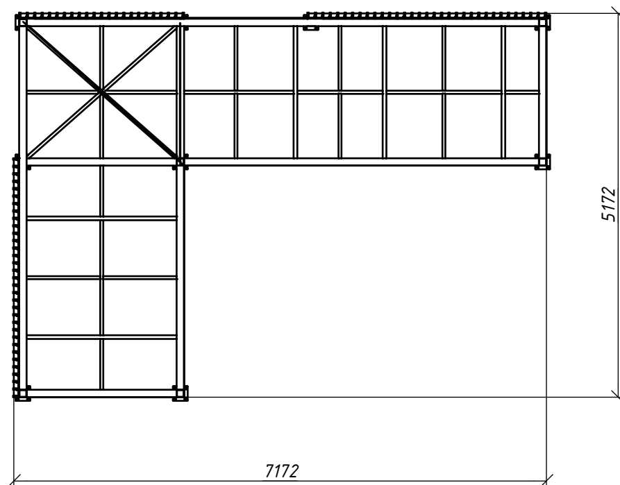
Вид зверху ( 1 : 50 )
