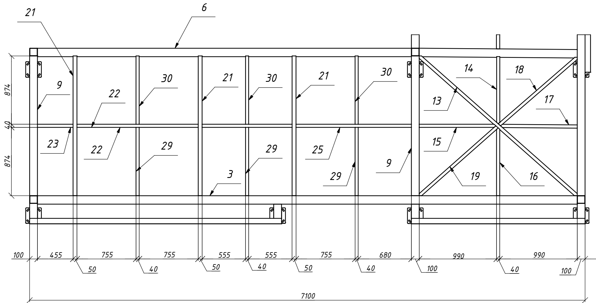
План покрівлі ( 1 : 20 ) 1ч.
