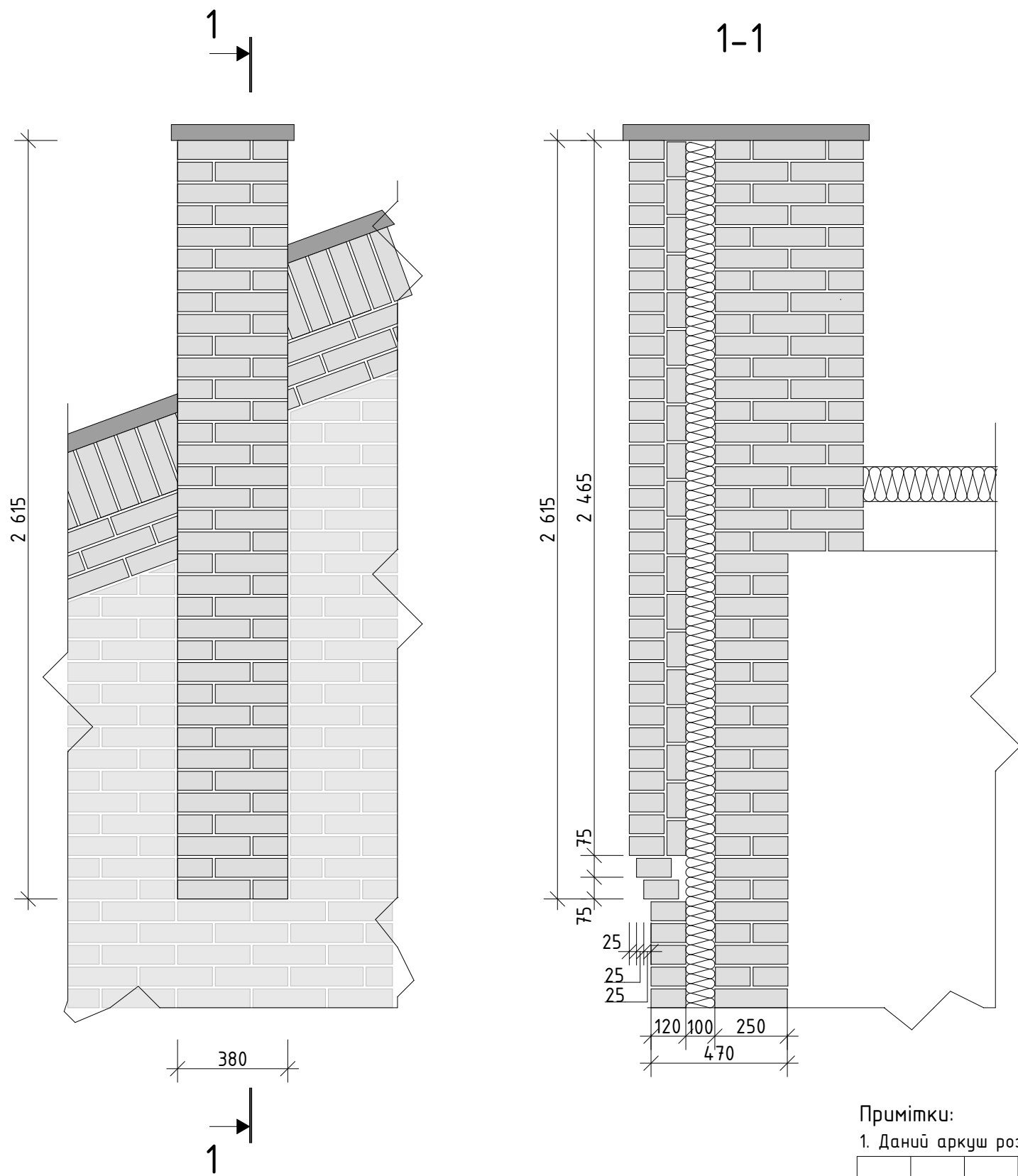
Вузол 5
