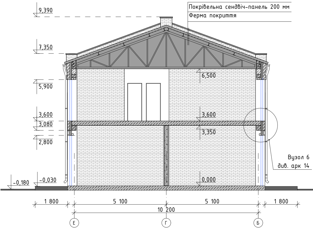
Розріз 2-2
