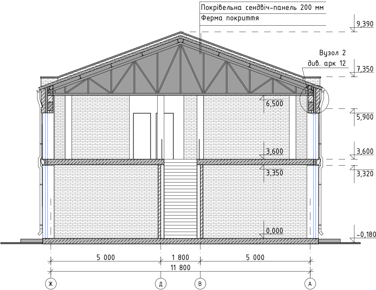
Розріз 3-3
