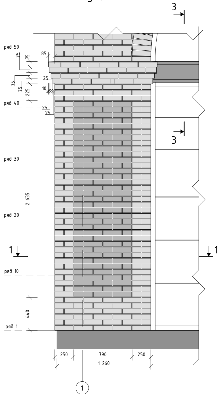
Вузол 4
