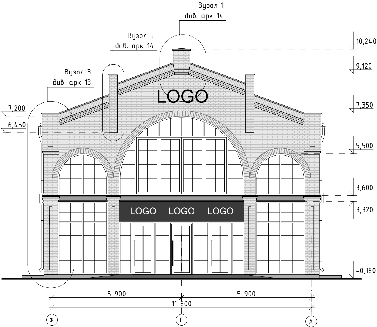
Фасад Ж-А
