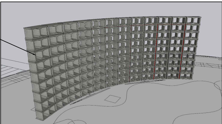
Стіна Б
