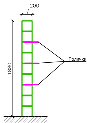
Розріз 1-1
