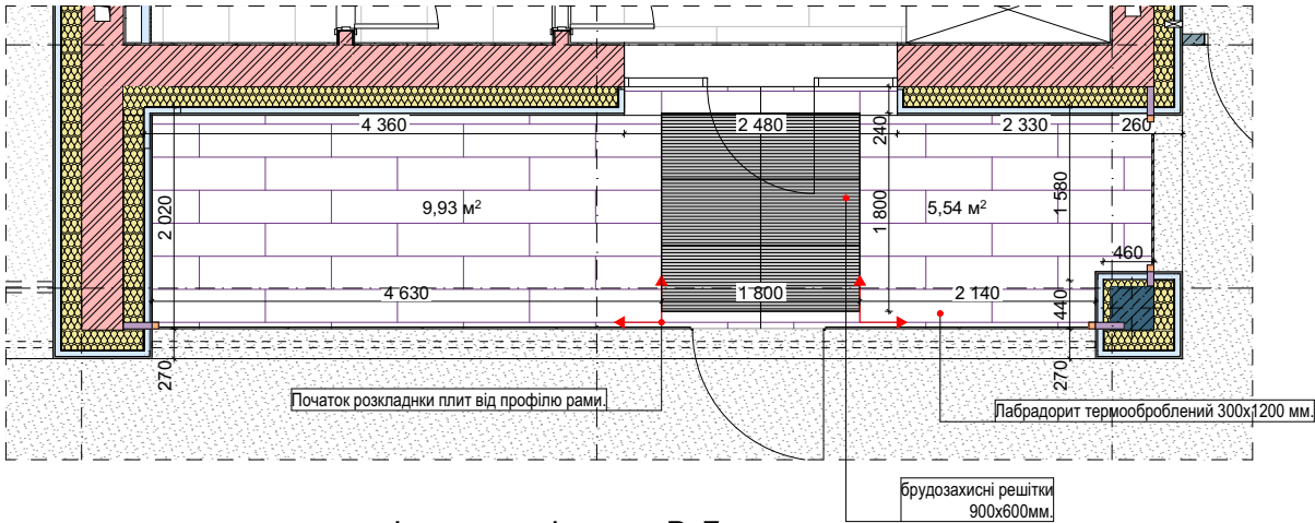
Фрагмент фасаду В-Д
