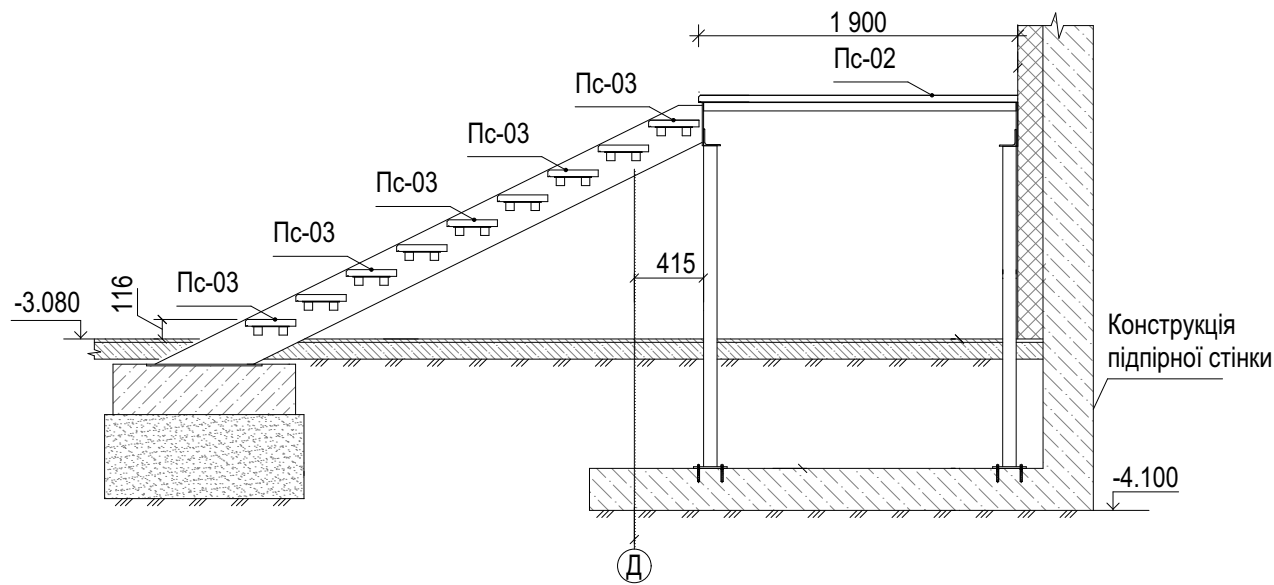
Розріз 3-3
