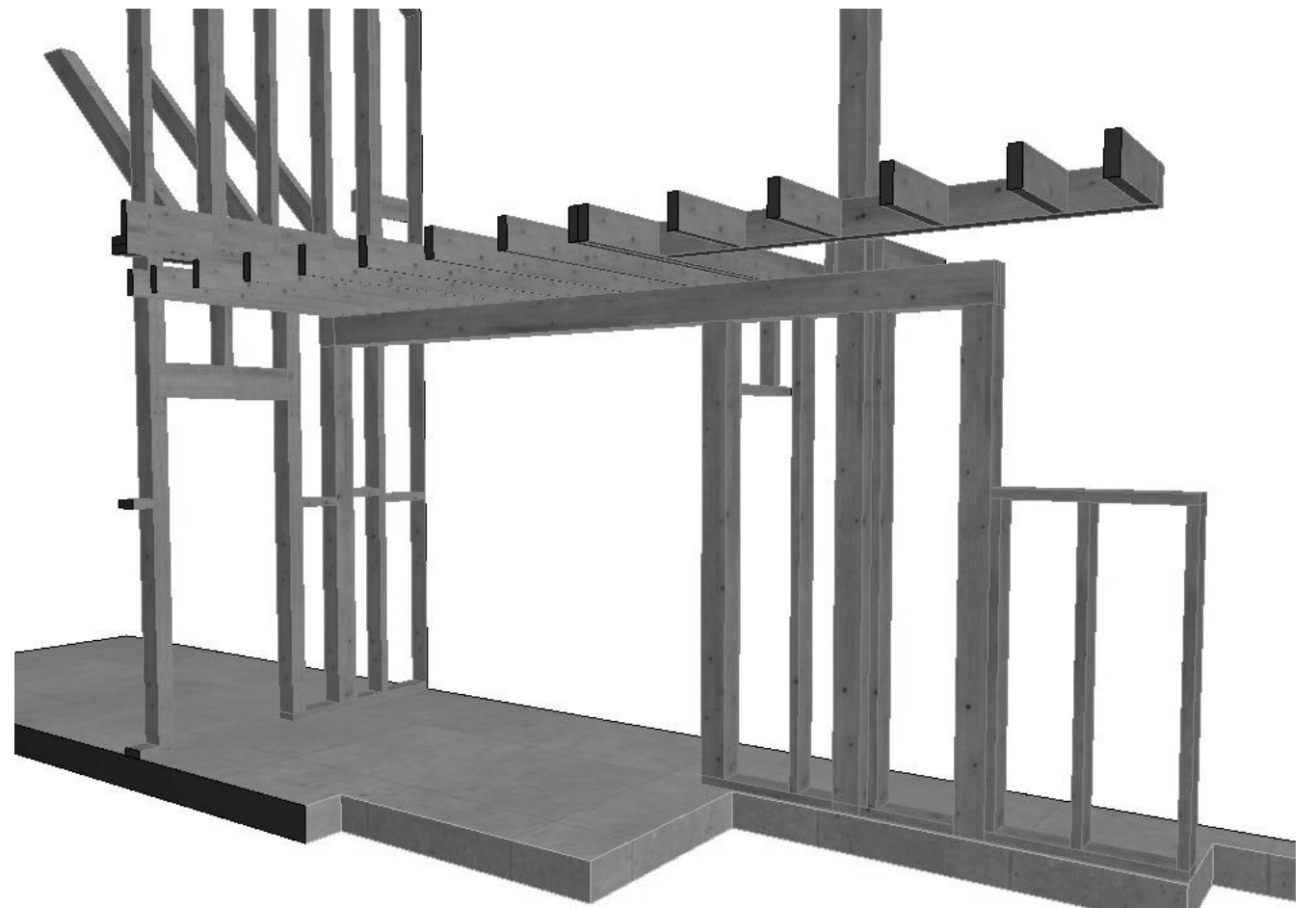
Фронтон Ф1 2x50x150 50x150 50x200 2x50x150 50x100 3x50x150 50x150 50x150 3x50x200 3x50x150 50x150 50x150 50x150 150 3 000 150 450 200 150 495 150 400 400 50 50 50 1 590 50 2 550 200 2 950 100 200 100 2 050 150 2 950 150
