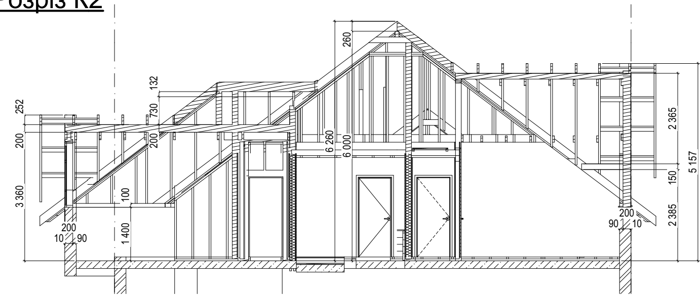
Розріз К2
