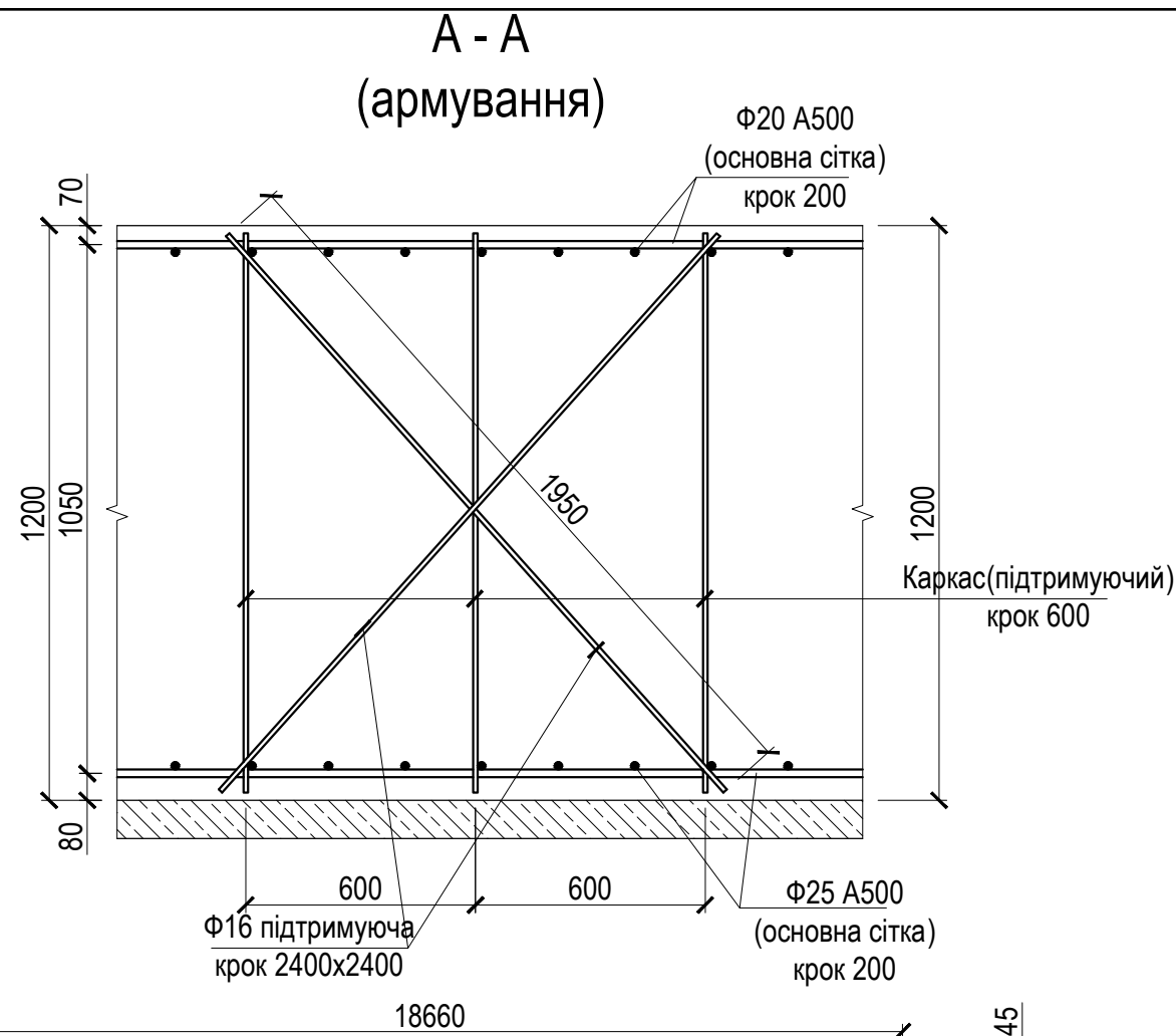
Схема розташування ростверку. Секція "Б".
