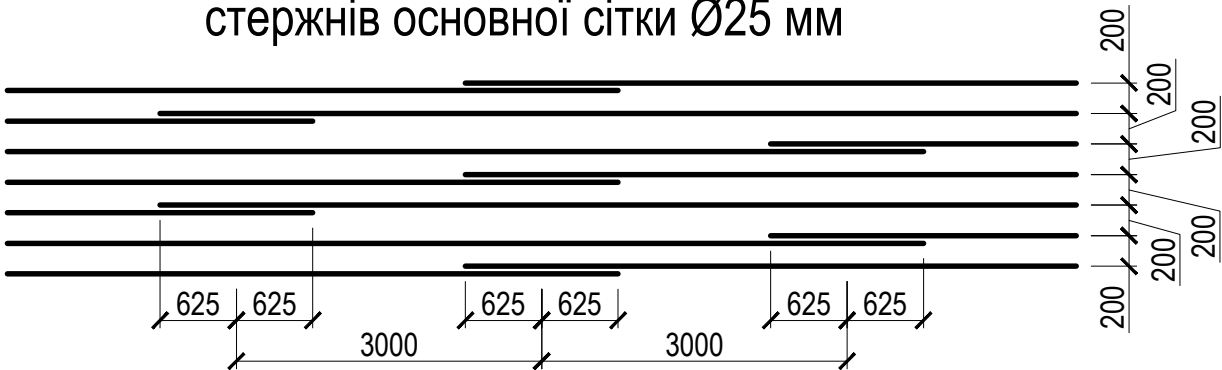
Деталь стикування перепуском арматурних стержнів основної сітки Ø25 мм
