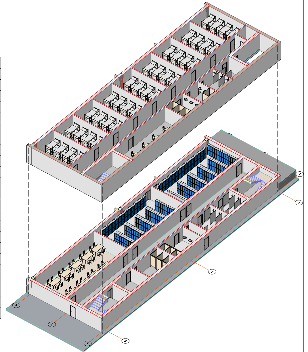
№ п/п пов. Найменування Площа, м 2 01 1 Їдальня 67,15 02 1 Роздягальня Ж 61,80 03 1 Душова Ж 12,60 04 1 Роздягальня М 63,64 05 1 Душова М 11,26 06 1 Санвузол М 15,44 07 1 Санвузол Ж 15,44 08 1 Технічне приміщення 11,27 09 2 Спальня 1 22,91 10 2 Спальня 2 23,16 11 2 Спальня 3 23,16 12 2 Спальня 4 23,16 13 2 Спальня 5 23,16 14 2 Спальня 6 23,16 15 2 Спальня 7 23,16 16 2 Спальня 8 23,16 17 2 Спальня 9 24,78 18 2 Кухня 31,72 19 2 Санвузол М 8,69 20 2 Санвузол Ж 10,38 21 2 Душова М 9,45 22 2 Душова Ж 9,22 23 2 Технічне приміщення 4,04
