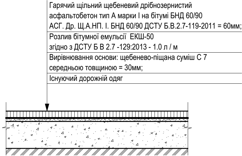
Конструкція покриття тротуарів, доріжок (тип III)
