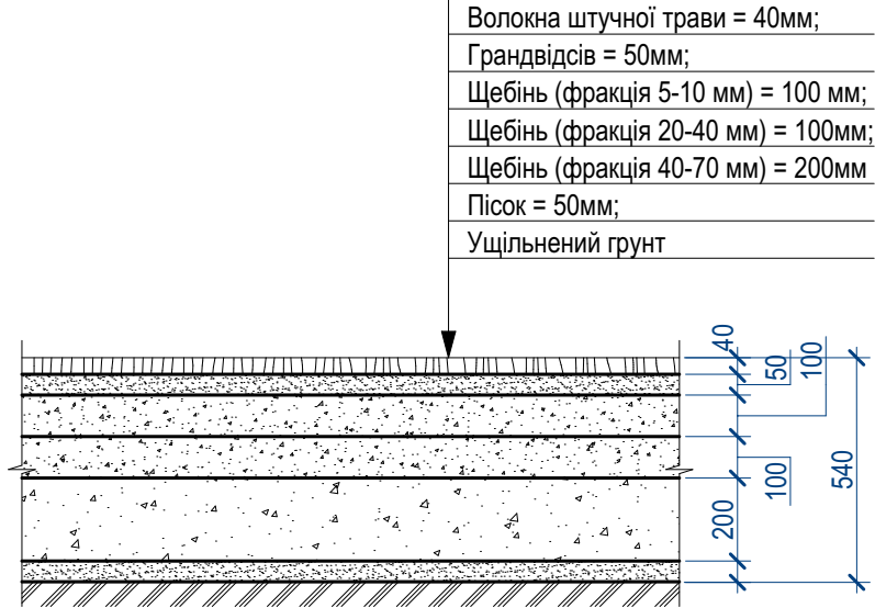
Конструкція покриття міні-футбольного поля (тип V)
