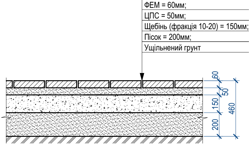
Конструкція покриття міні-футбольного поля (тип V)
