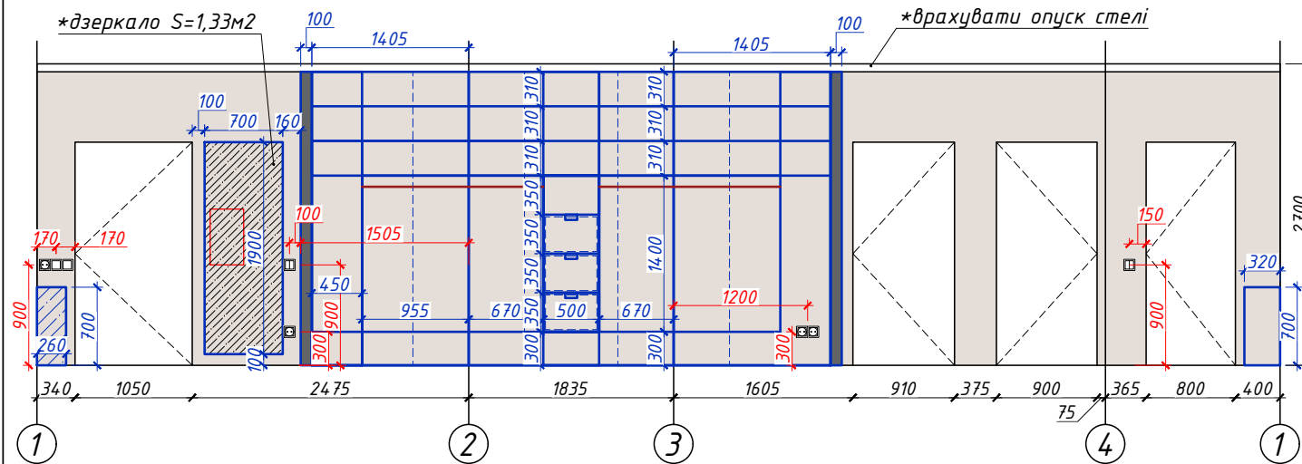
Фрагмент плану
