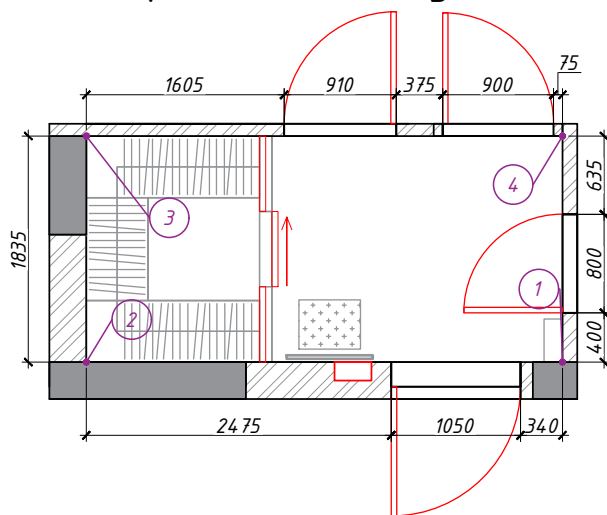
Фрагмент плану
