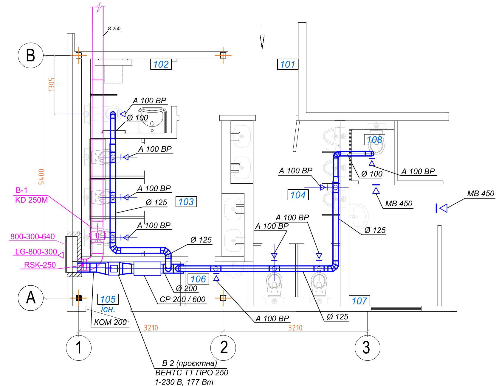
План монтажу проеткної системи вентиляції м 1:50
