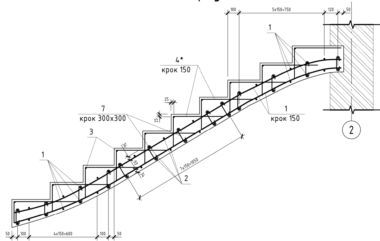
С4-С4 (Армування)
