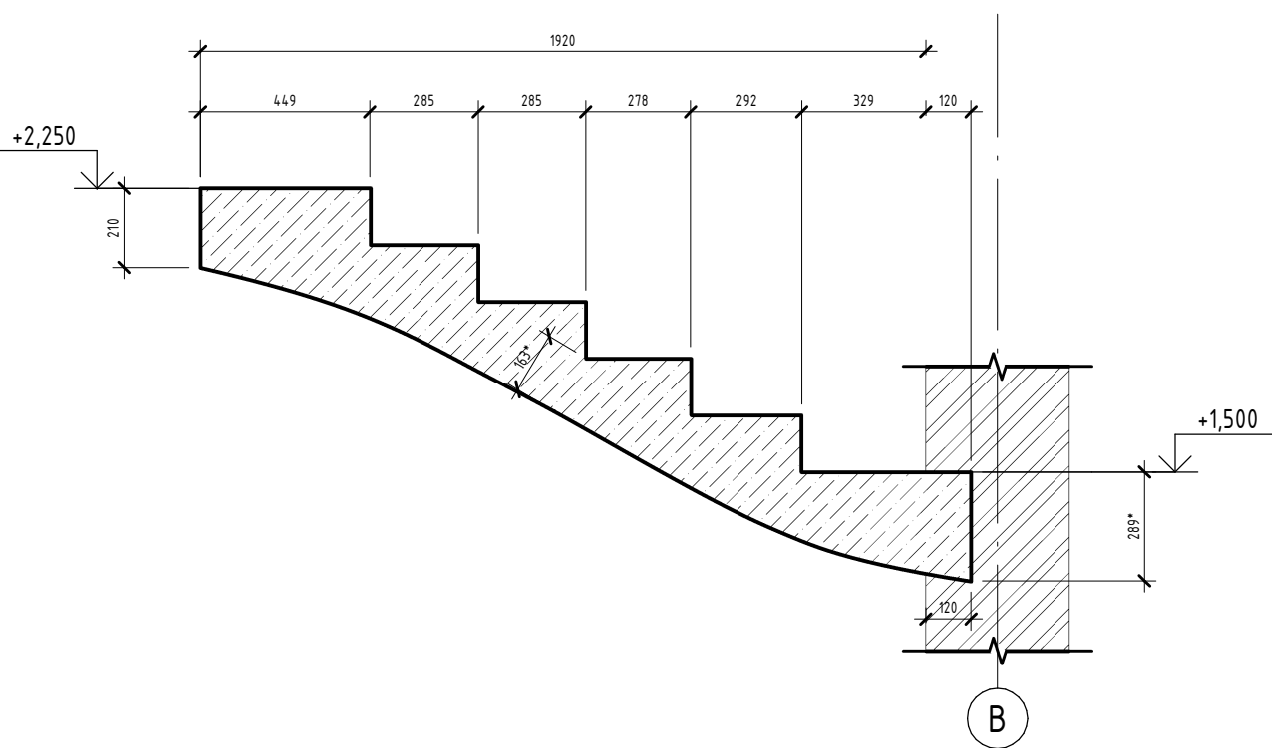
С5-С5 (Опалубка)
