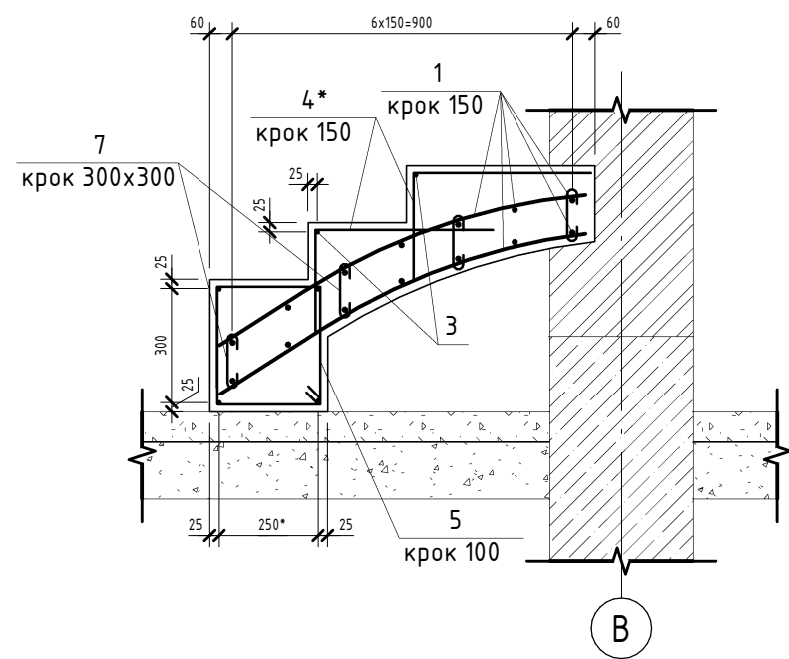
С3-С3 (Армування)
