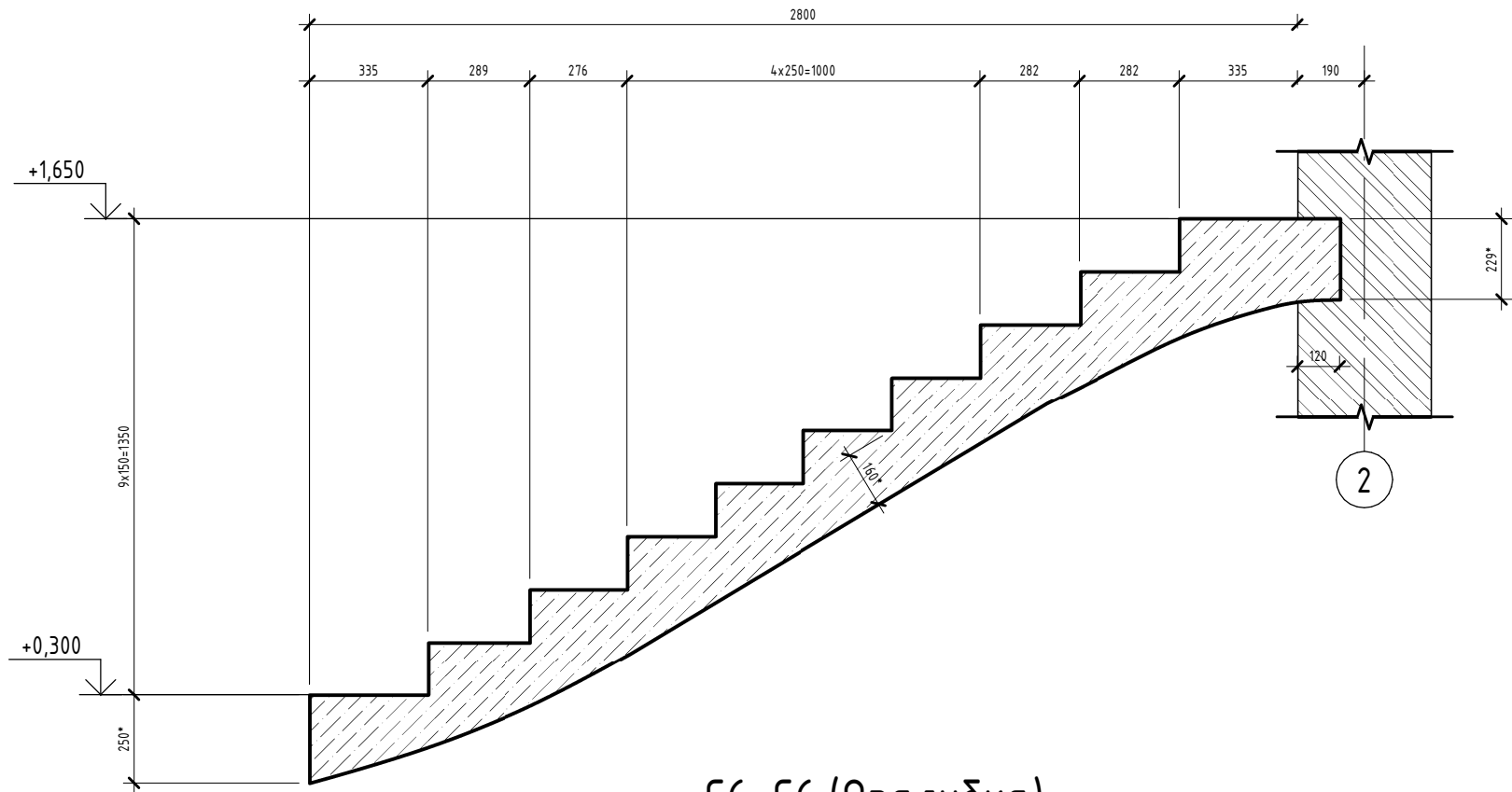
С6-С6 (Опалубка)
