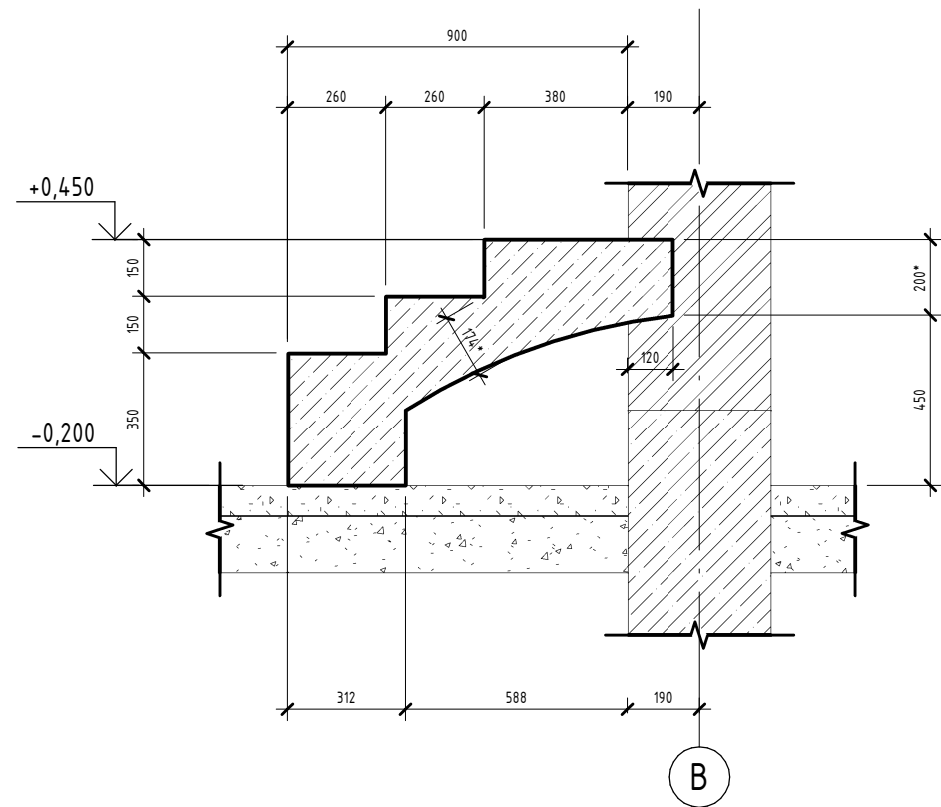
С5-С5 (Опалубка)
