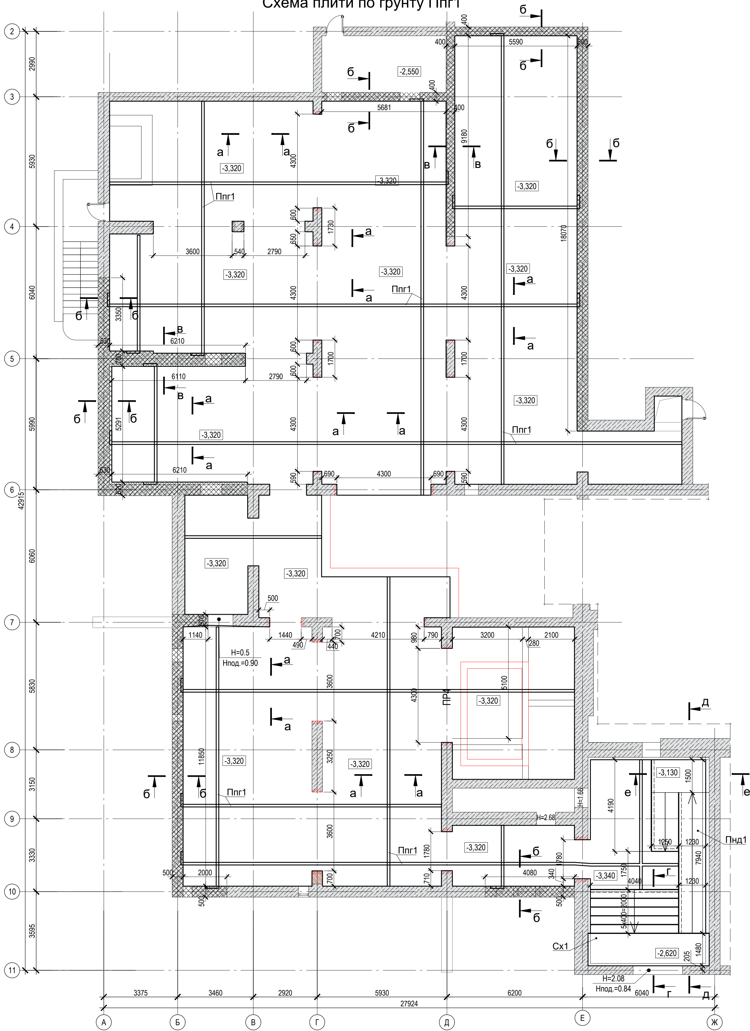
Схема плити по ґрунту Пгр1
