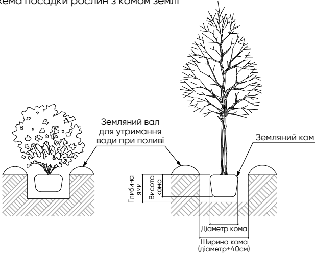
Схема посадки рослин з комом землі
