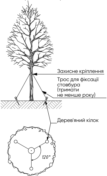
Схема кріплення дерев після посадки
