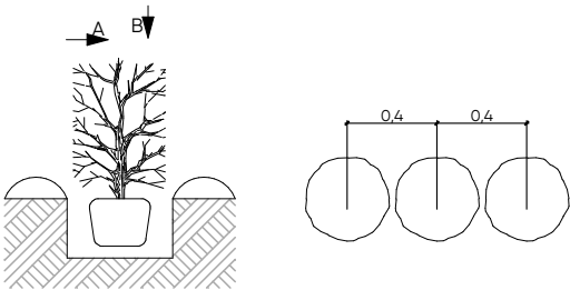
Схема посадки живоплоту з чагарників з комом землі
