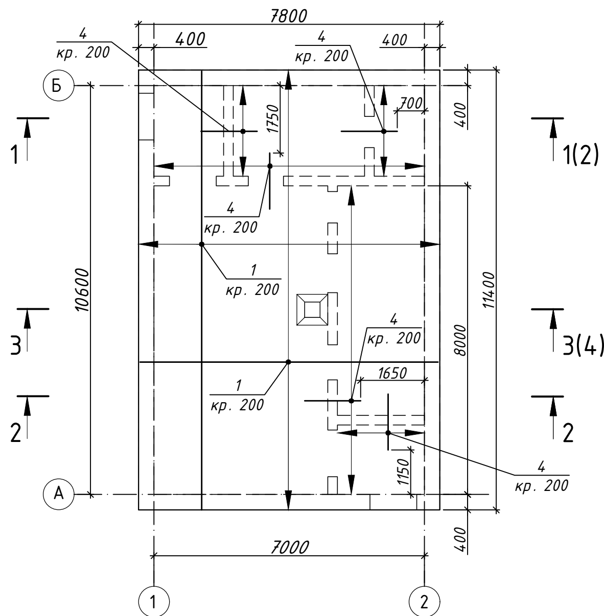
Плита фундаментна ПФМ1 Схема розташування нижньої арматури
