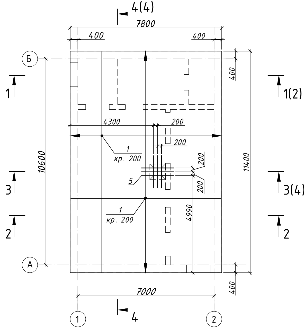
Плита фундаментна ПФМ1 Схема розташування верхньої арматури
