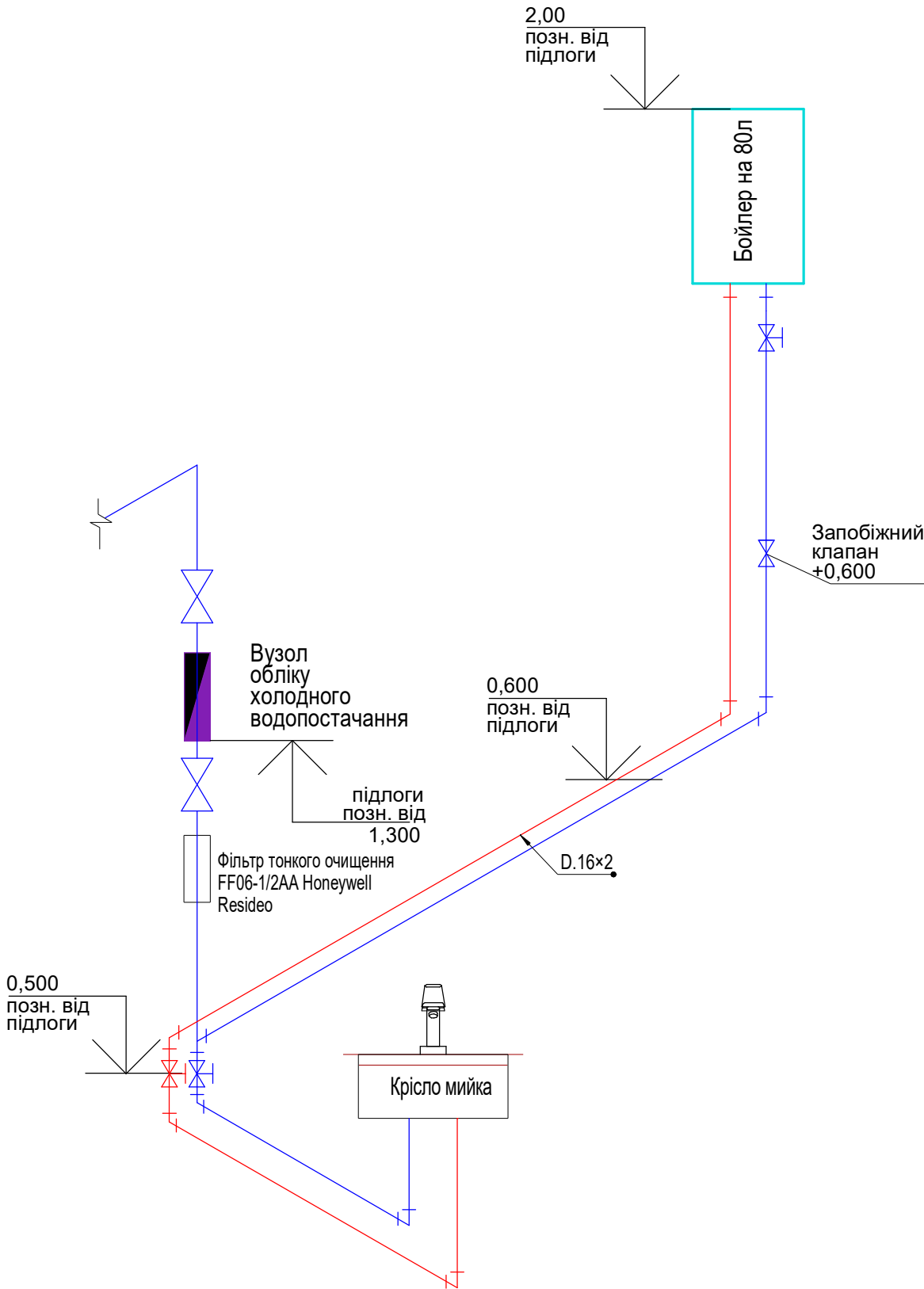
Схема підключення водопроводу
