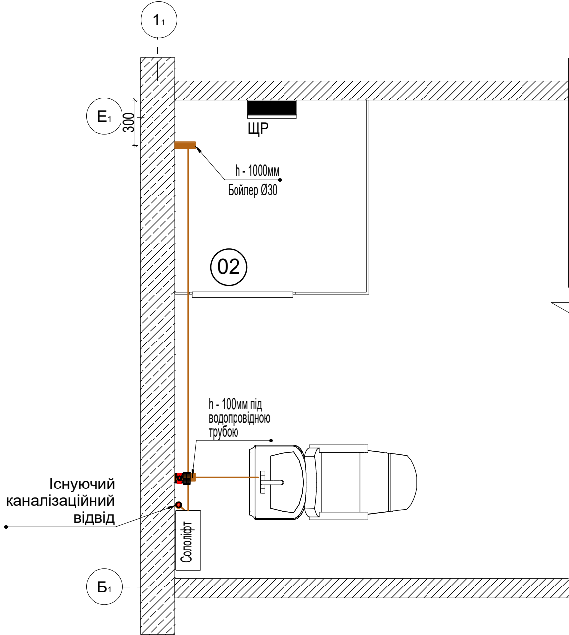
План з розміщенням каналізації масштаб 1:40
