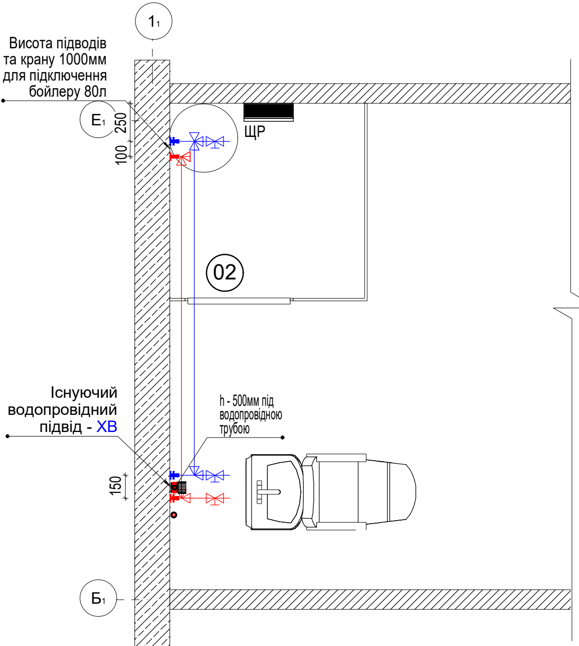
План з розміщенням водопроводу масштаб 1:40
