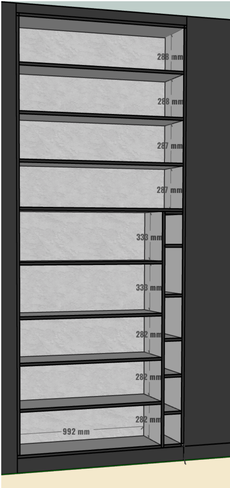
ніша та частина шафи у розрізі з розмірами
