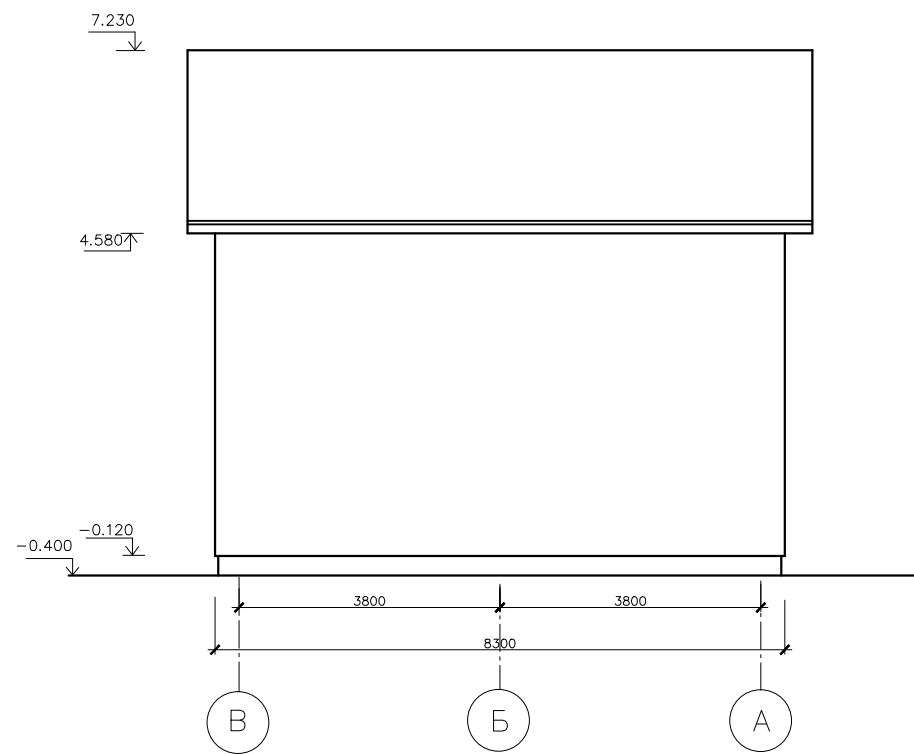
Фасад в осях В—А
