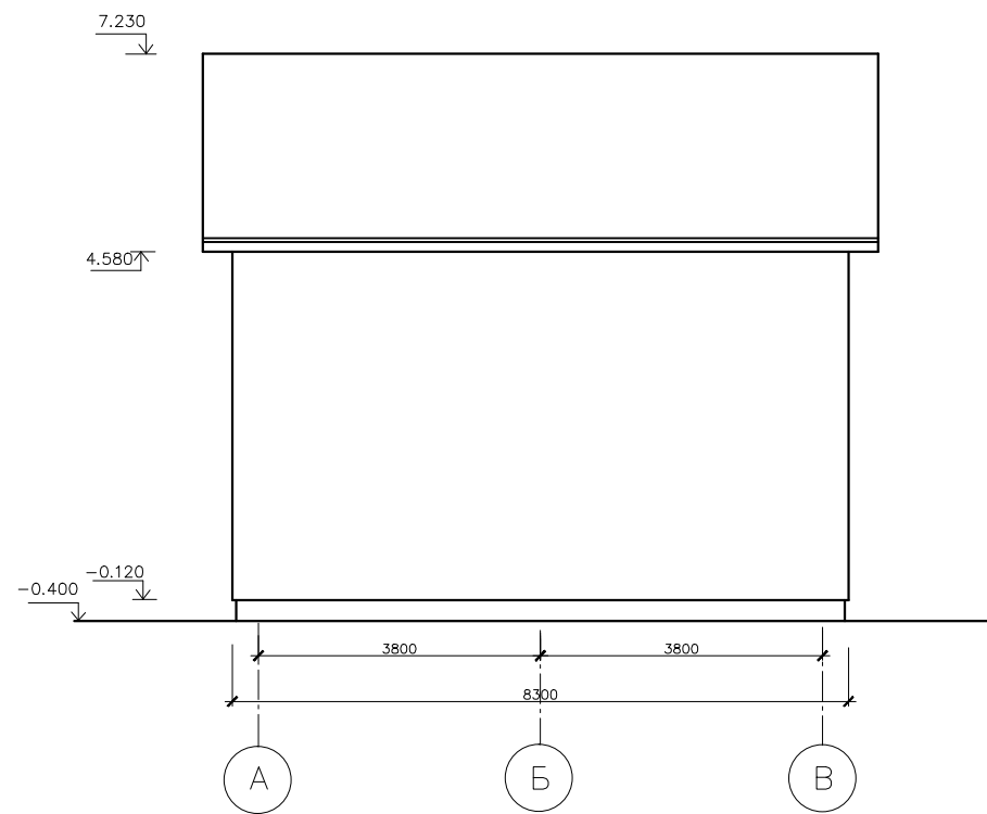
Фасад в осях А—В
