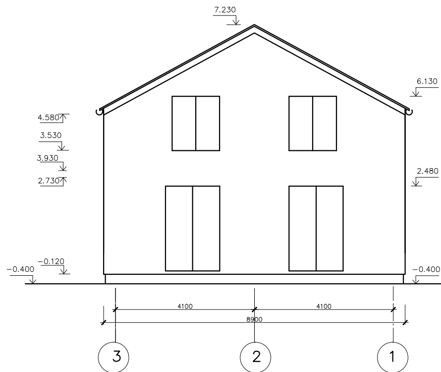
Фасад в осях 3—1
