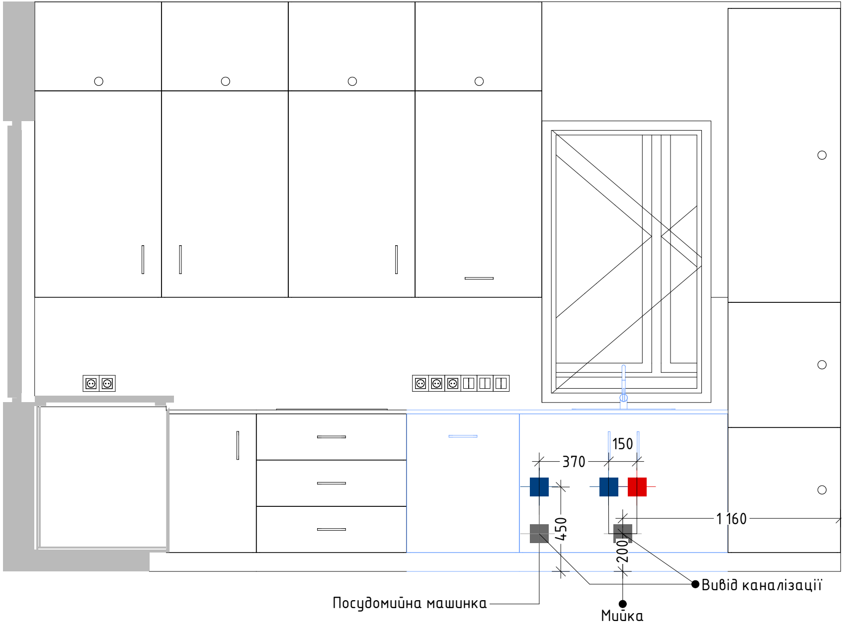
Розгортка 2.1
