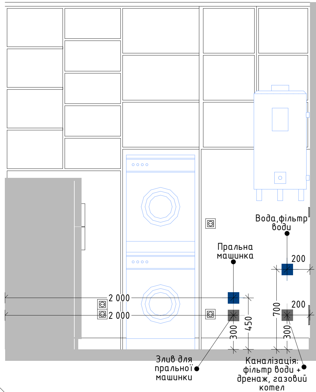
Розгортка 3.1
