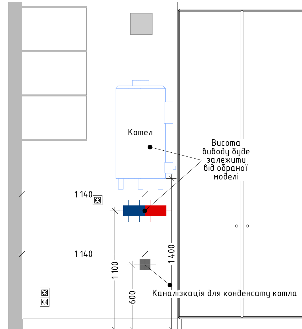
Розгортка 3.2
