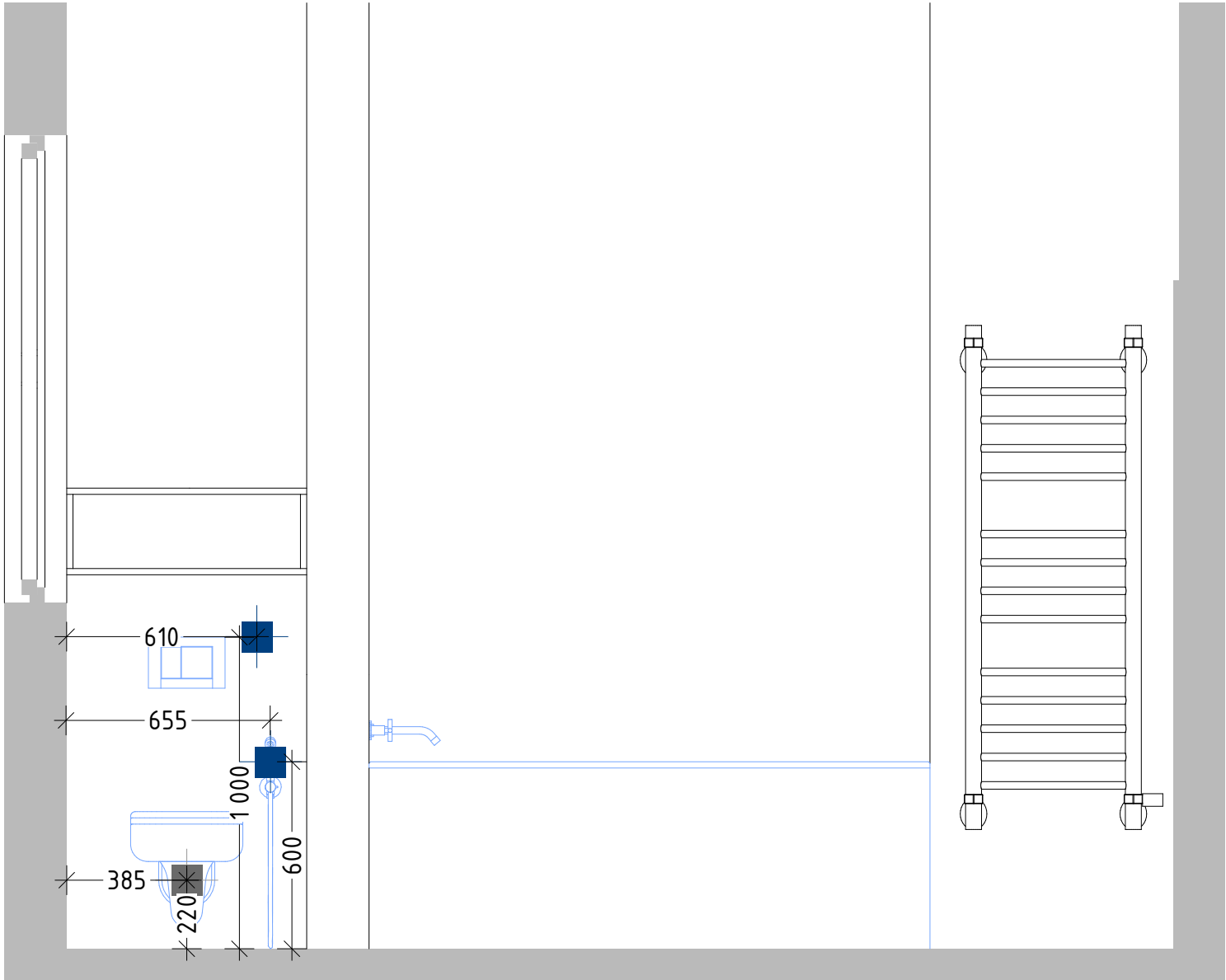
Розгортка 4.3
