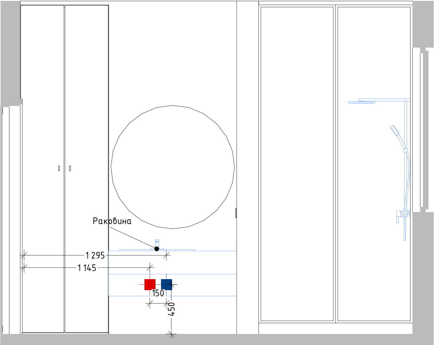
Розгортка 4.1
