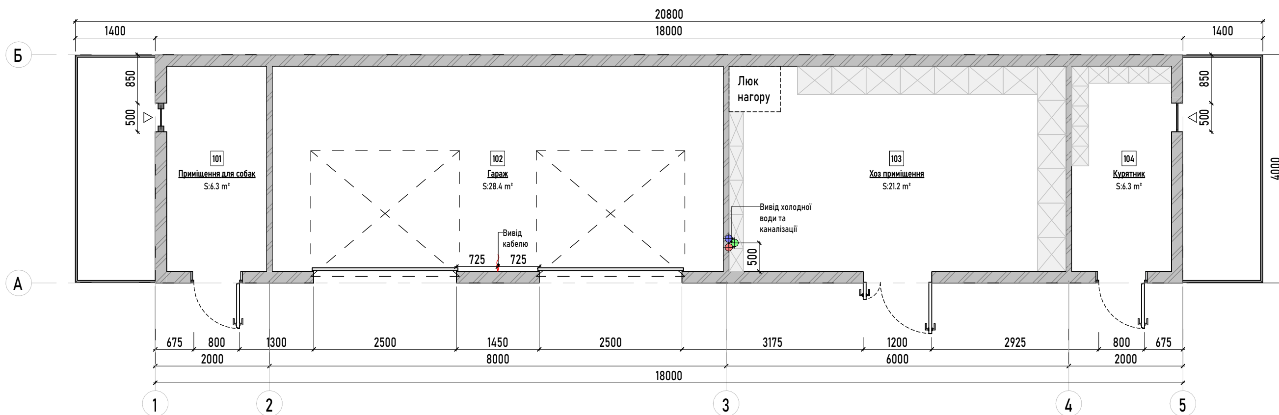
ПЛАН МЕБЛІВ ТА ОБЛАДНАННЯ М 1 : 65
