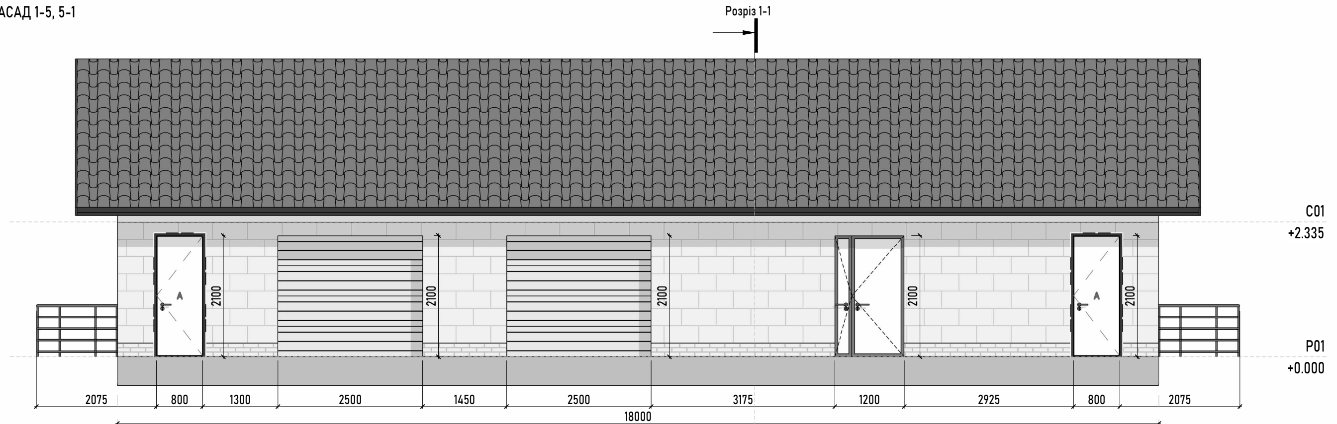
ФАСАД 1-5 М1:65
