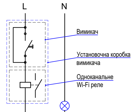
Схема підключення одноканального Wi-Fi реле
