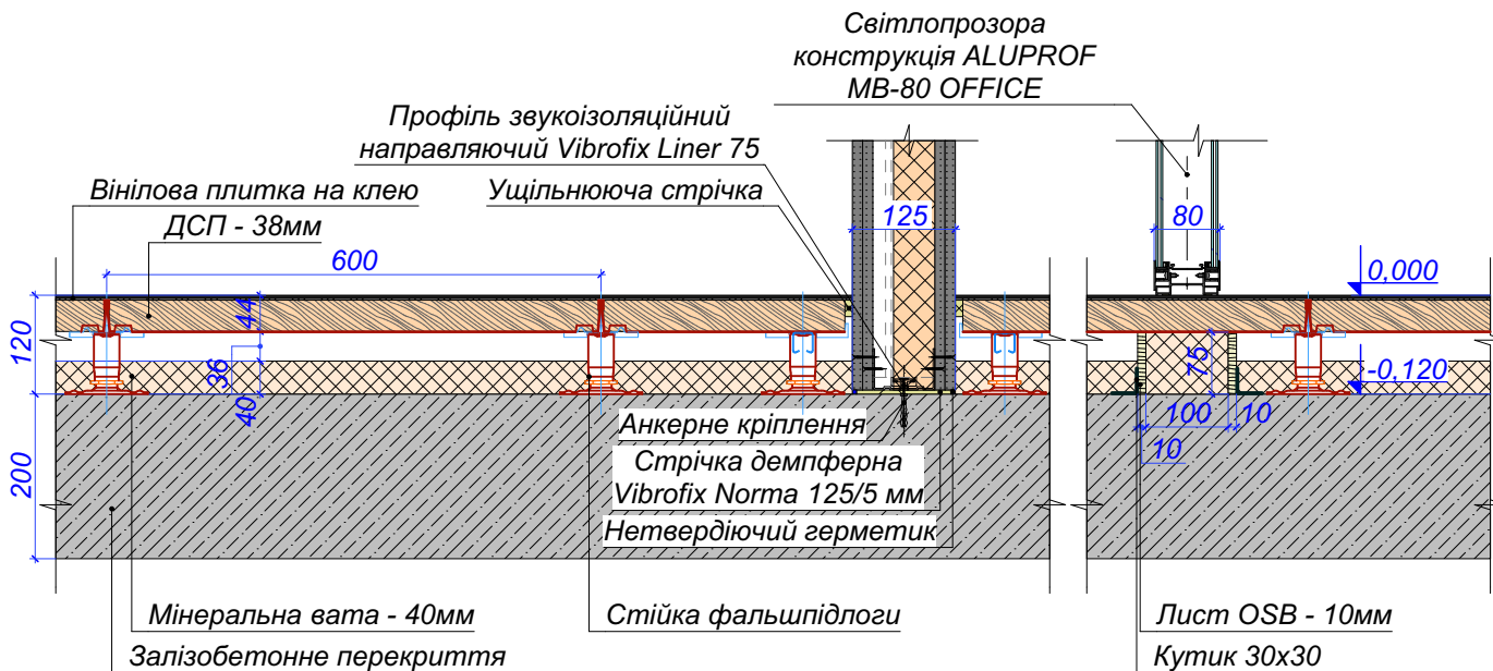
Вузол влаштування фальшпідлоги М 1:10
