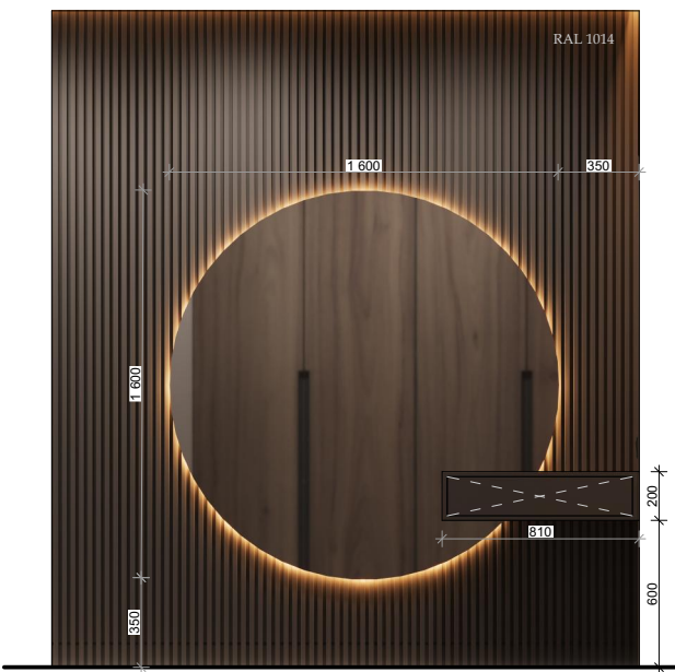
Розгортка B-B1
