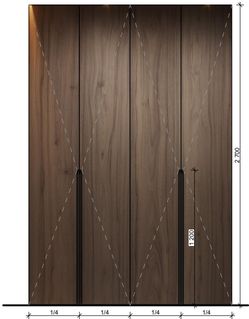
Розгортка A-A1
