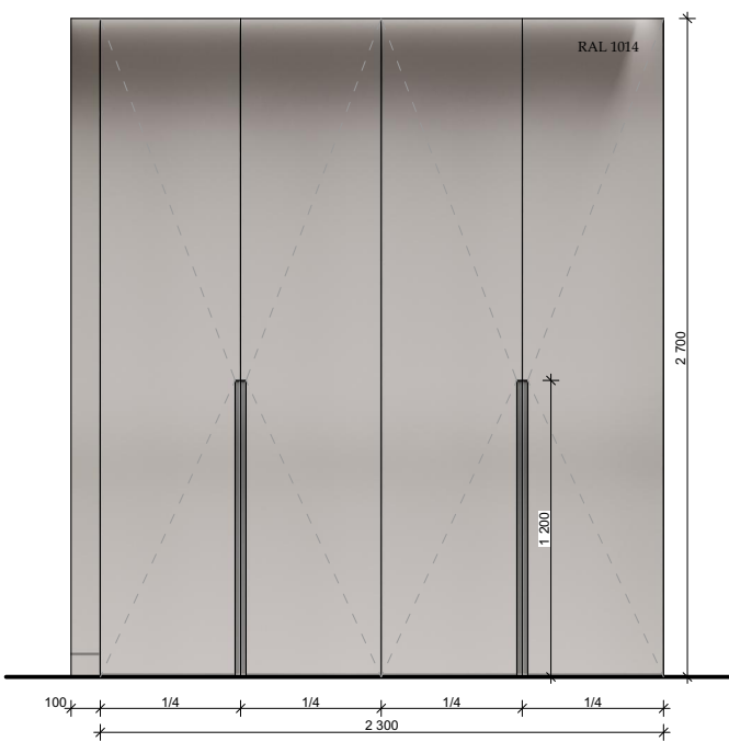
Розгортка J-J1
