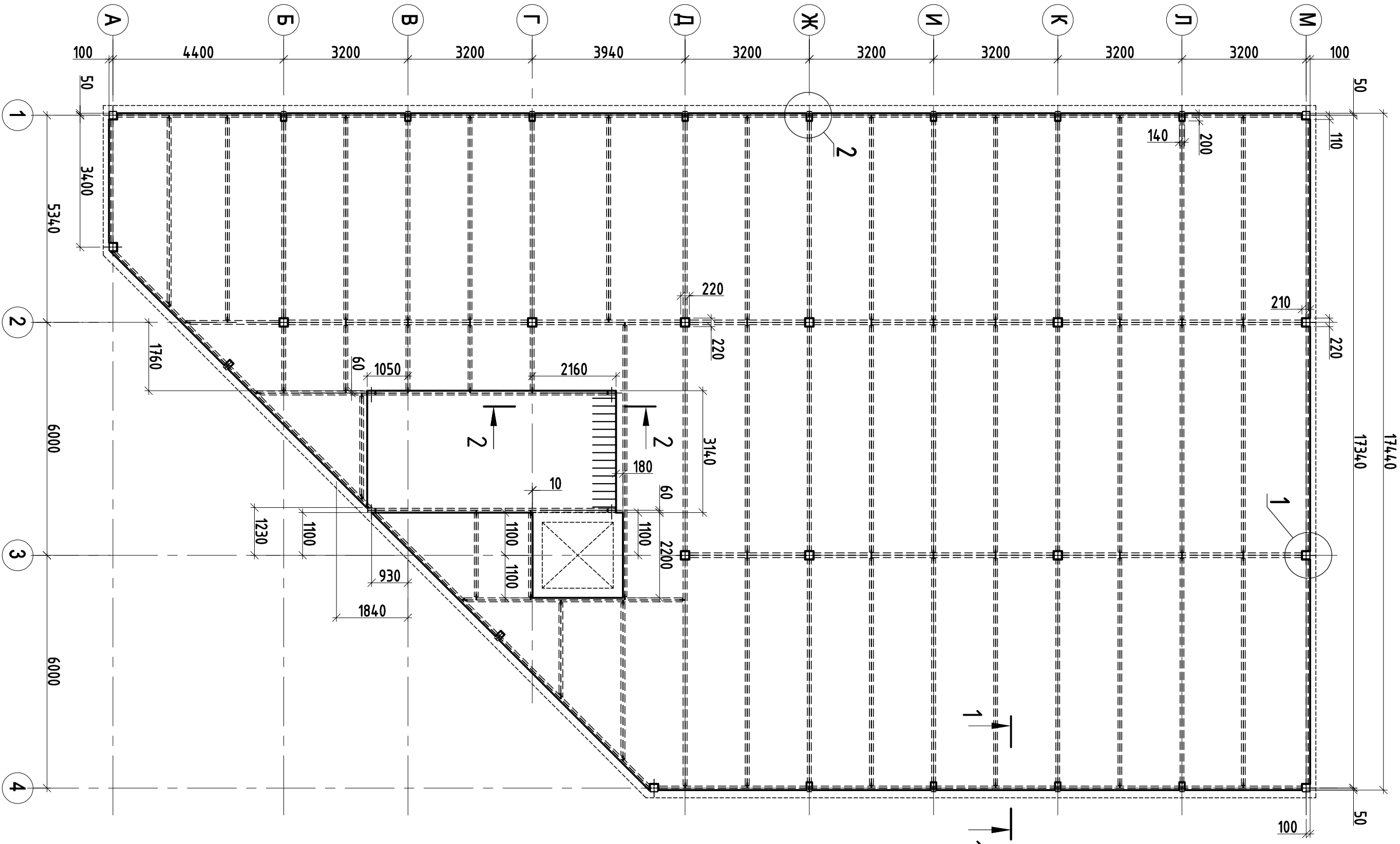
Схема розташування плити перекриття на відм. +3,300, +6,600, +9,900
