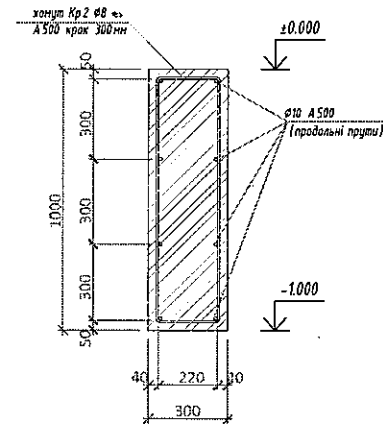
Переріз 1-1 (армування)
