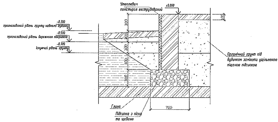
Переріз 1-1 (опалубочний) М 1:25
