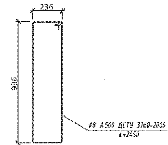
Каркас Кр1 380 шт.
