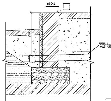
Переріз 3-3 точка виводу інженерних мереж (К1)
