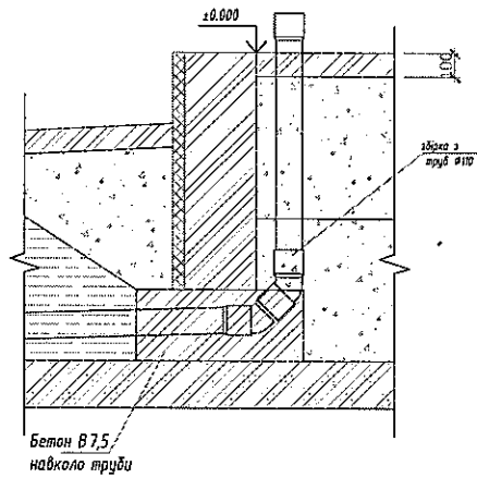
Переріз 2-2 точка вводу інженерних мереж
