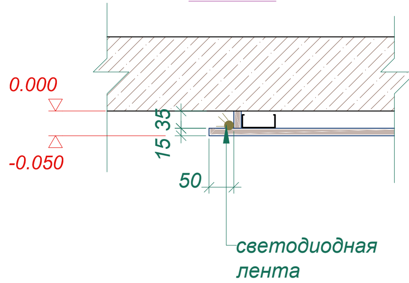
Узел Б
