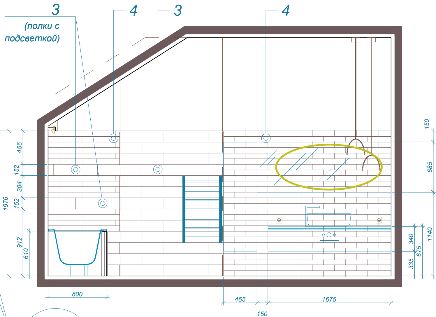
Разрез 2-2
