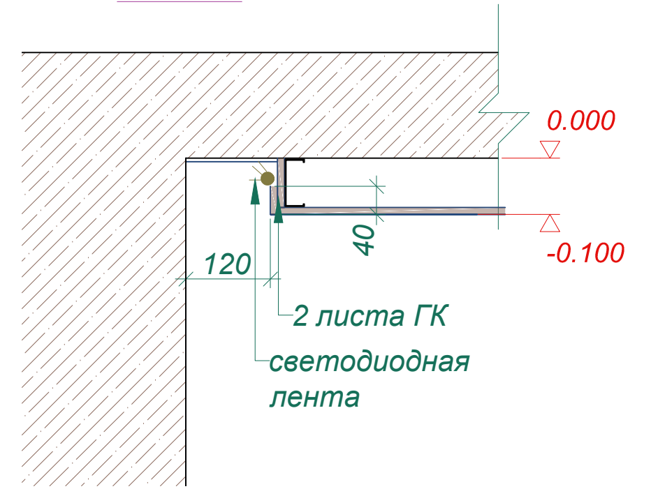
Узел В
