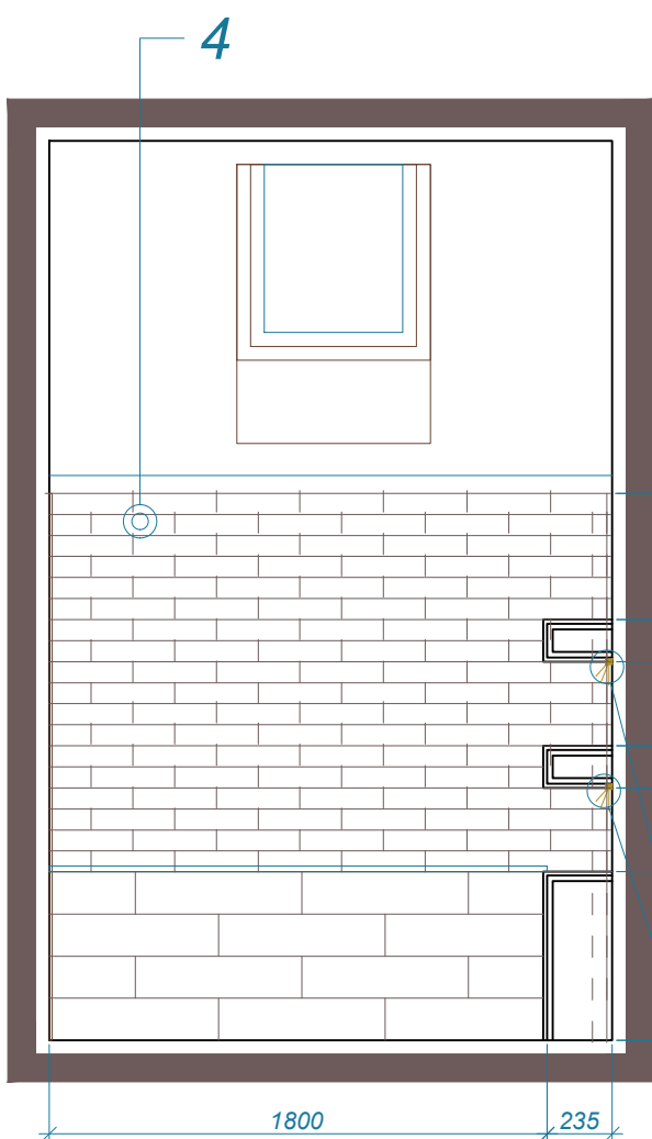
Разрез 1-1
