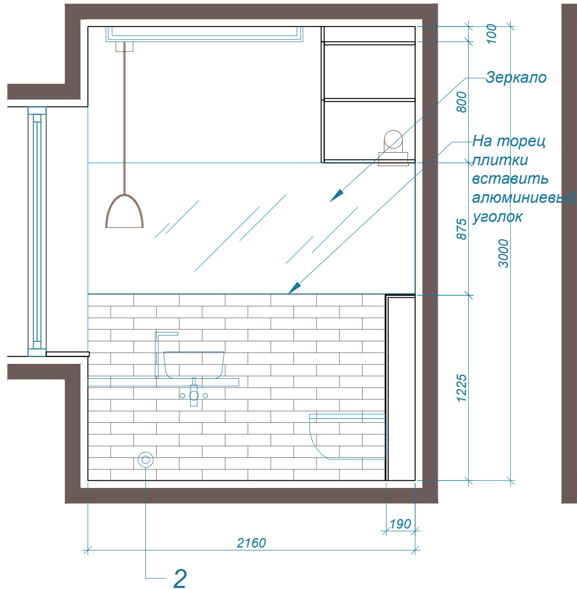
Разрез 1-1
