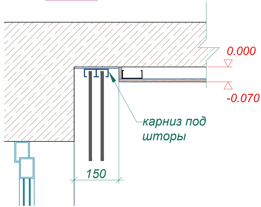
Узел Г
