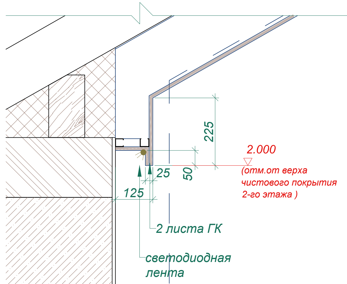
Узел Г
