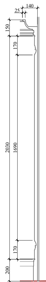
Сечение настенных панелей. М 1:20
