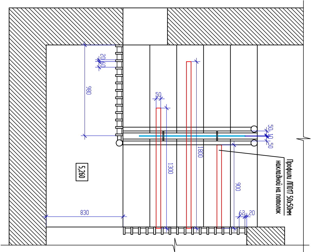
План верхней площадки
