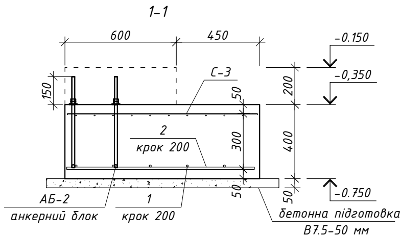
Деталь встановлення поз. 4 (армування фундаменту умовно не показано)
