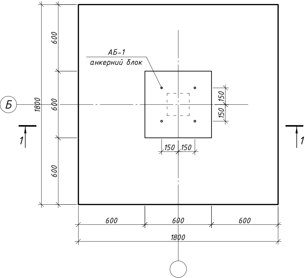
Фундамент ФМ-1
