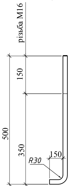
Шпилька анкерного болта (АБ-2, АБ-3)
