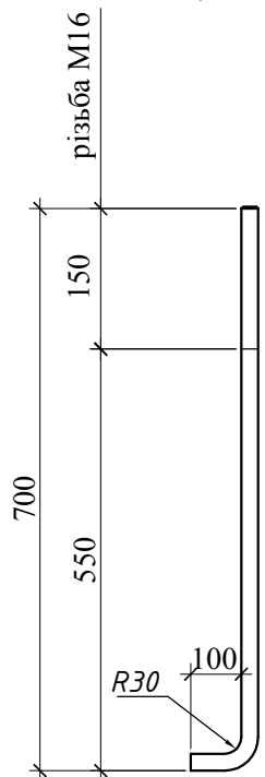
Шпилька анкерного болта (АБ-1)
