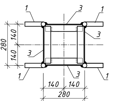
Анкерний блок АБ-3
