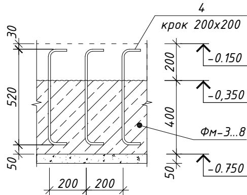
Деталь встановлення поз. 4 (армування фундаменту умовно не показано)
