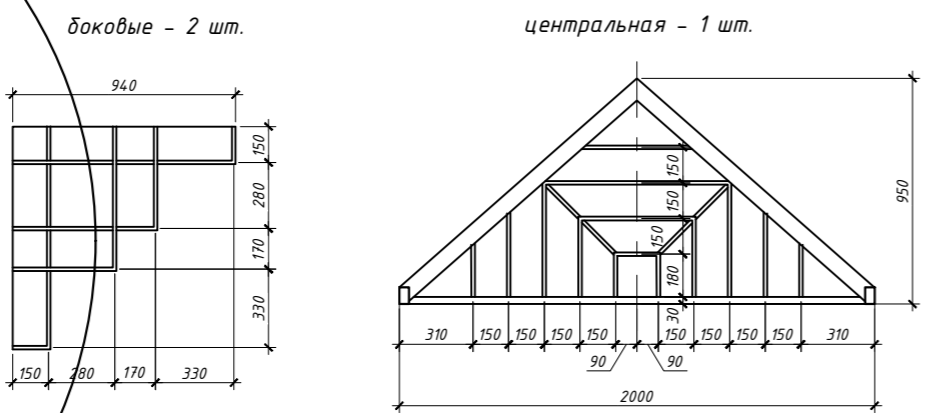
ЭСКИЗЫ РЕШЕТОК НАВЕСОВ НАД КРЫЛЬЦАМИ М 1:20
