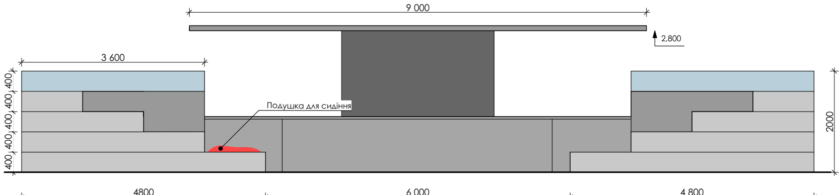
Вид А
