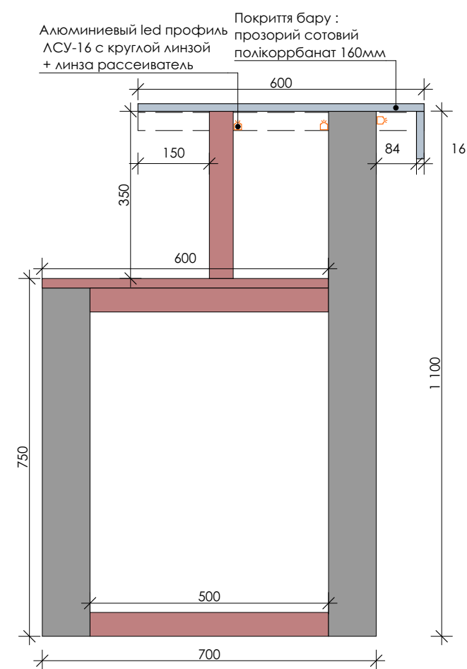
Розріз 2-2
