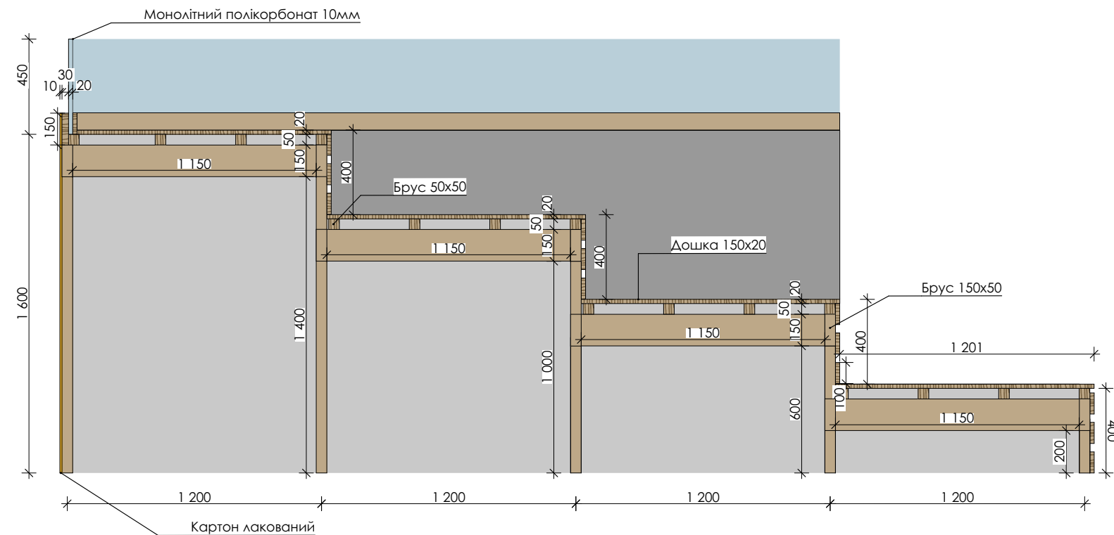
Розріз 1-1
