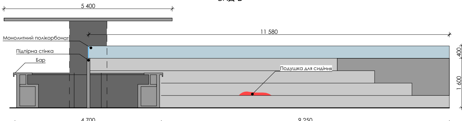
ВИД Б
