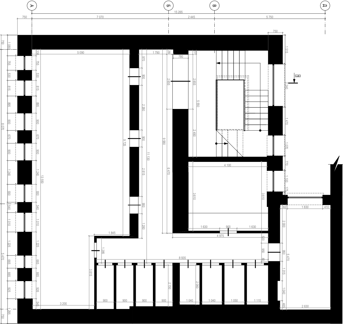
План 3-го поверху на відм. +7,500
