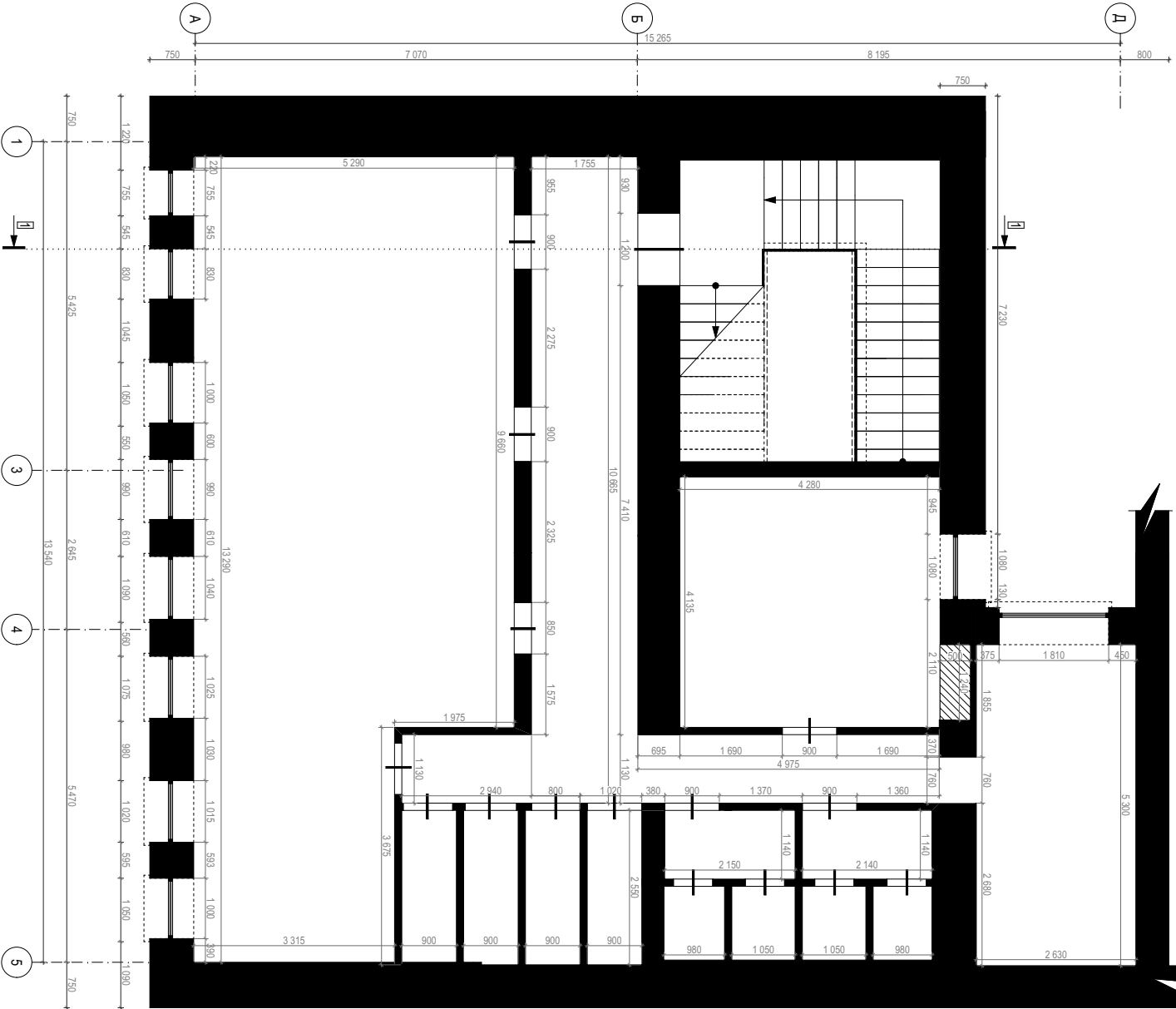
План 2-го поверху на відм. +4,000
