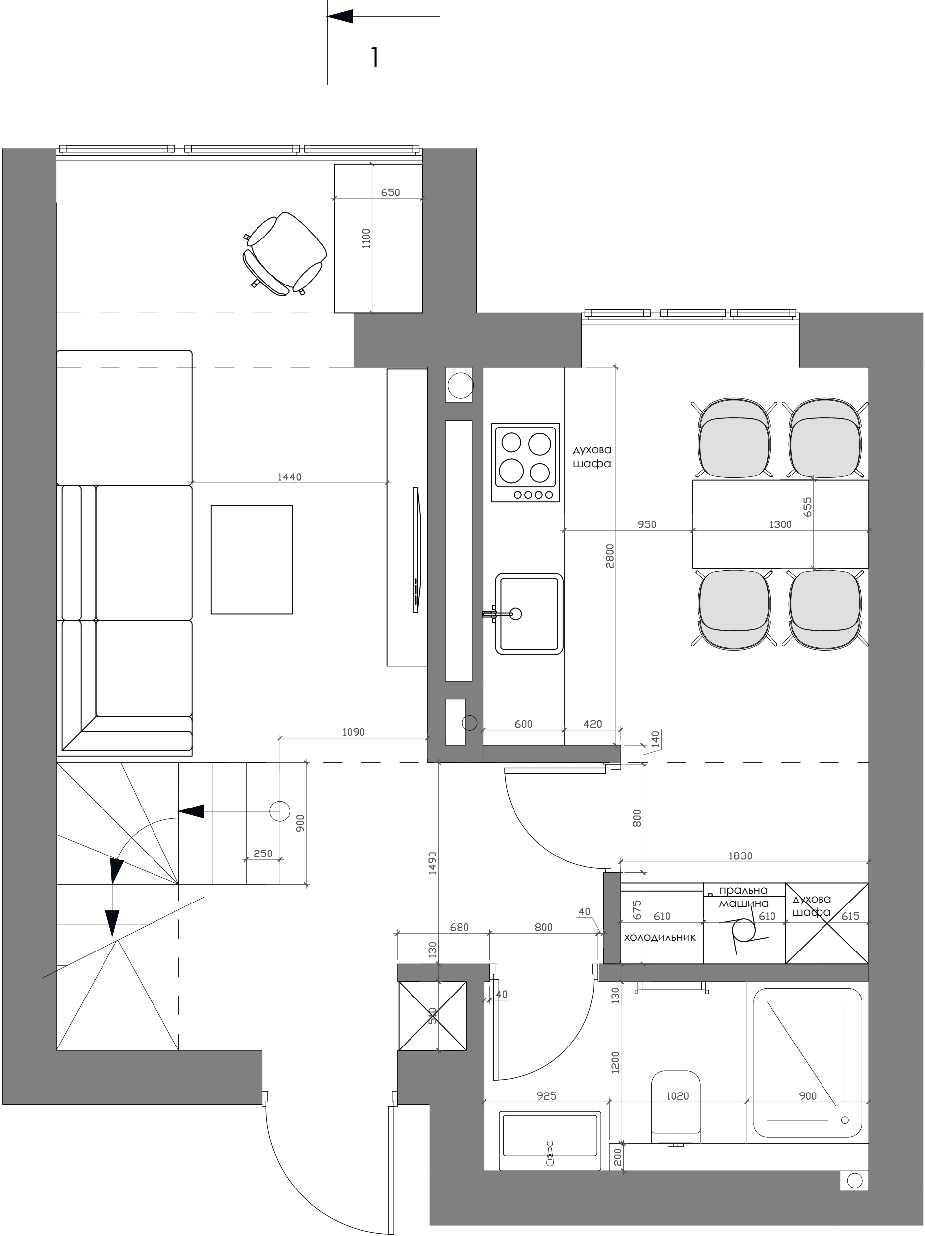
План на відмітці +0,000
