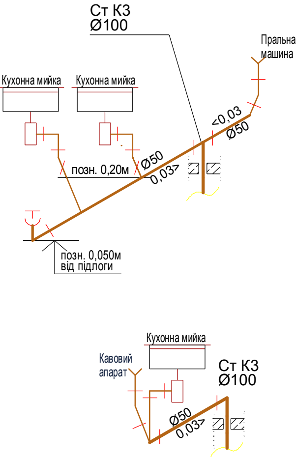
Схема підключення каналізації
