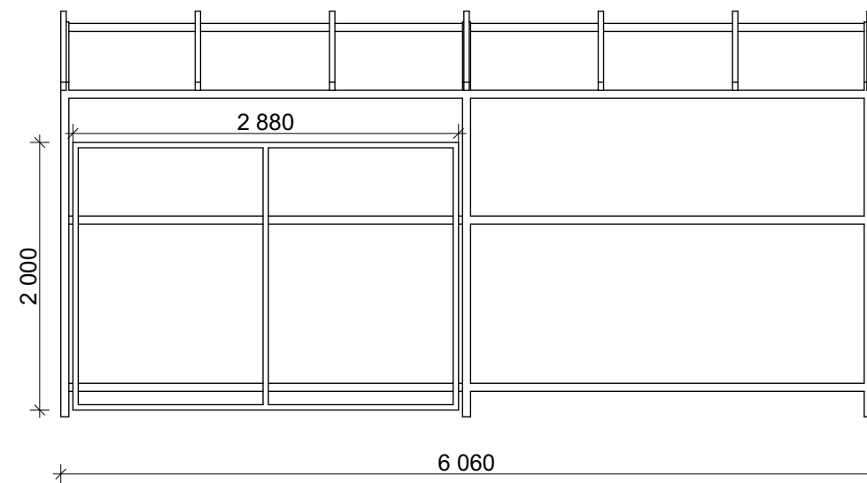
Розріз 2-2 М 1:50
