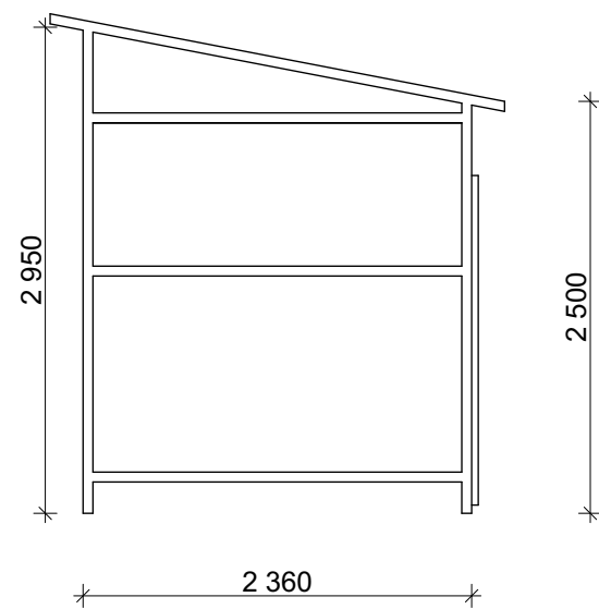
Розріз 1-1 М 1:50
