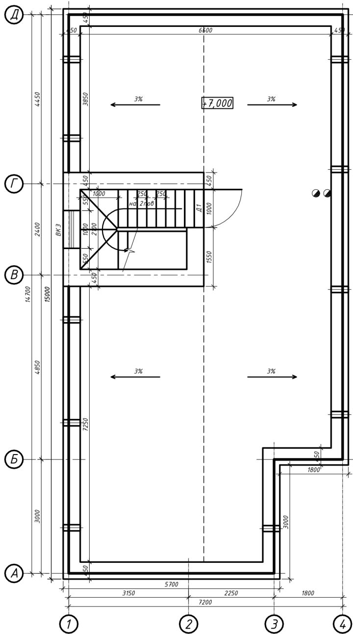
План даху на відм. +7,000
