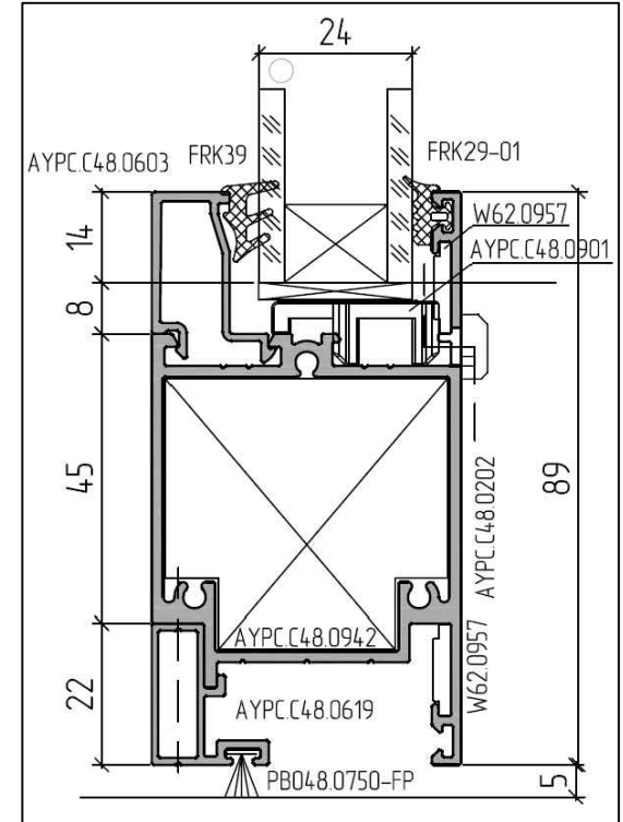
Розріз 1-1
