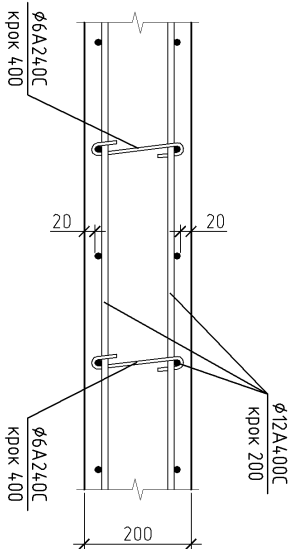
Вузел Б
