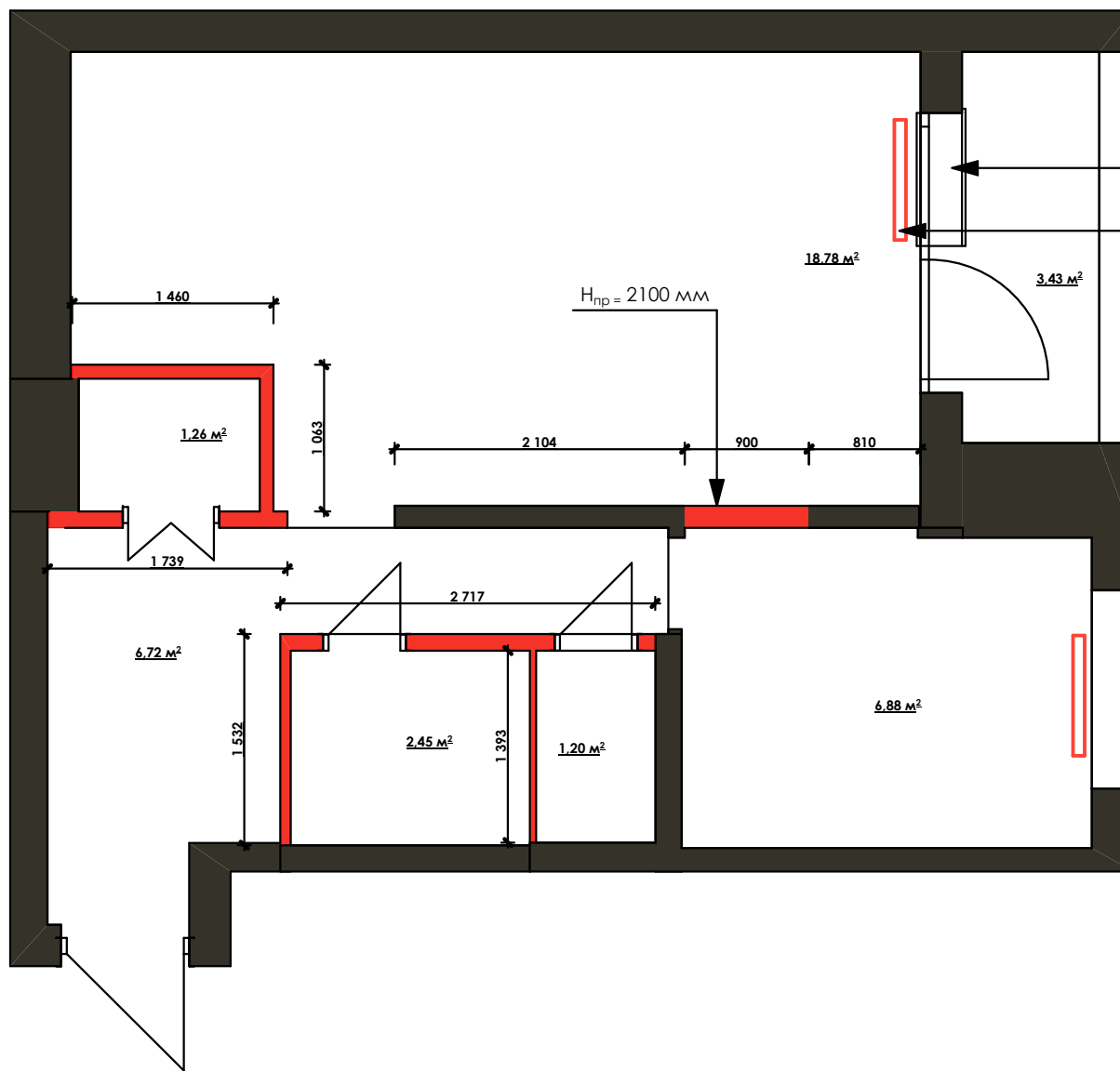
ПЛАН ДЕМОНТАЖА М 1:100
