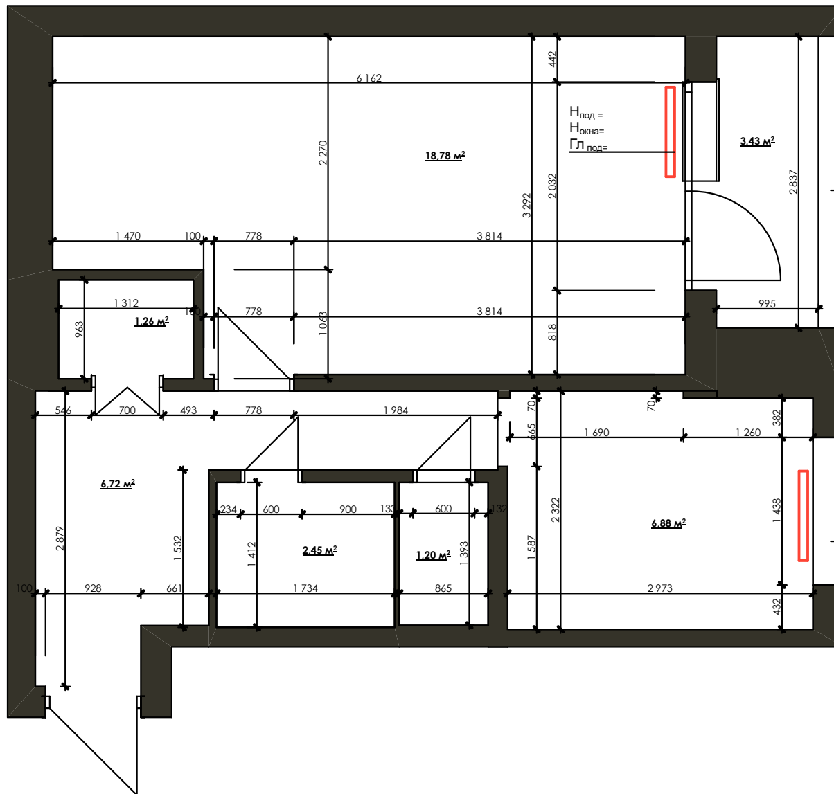
ПЛАН ОБМЕРНЫЙ М 1:100
