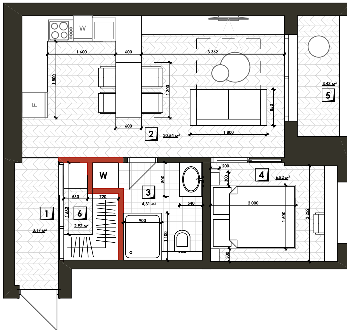
ПЛАН ПЕРЕПЛАНИРОВКИ М 1:100
