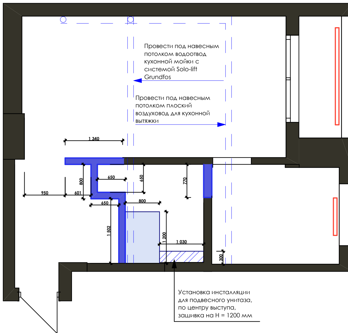
ПЛАН МОНТАЖА ПЕРЕГОРОДОК М 1:100
