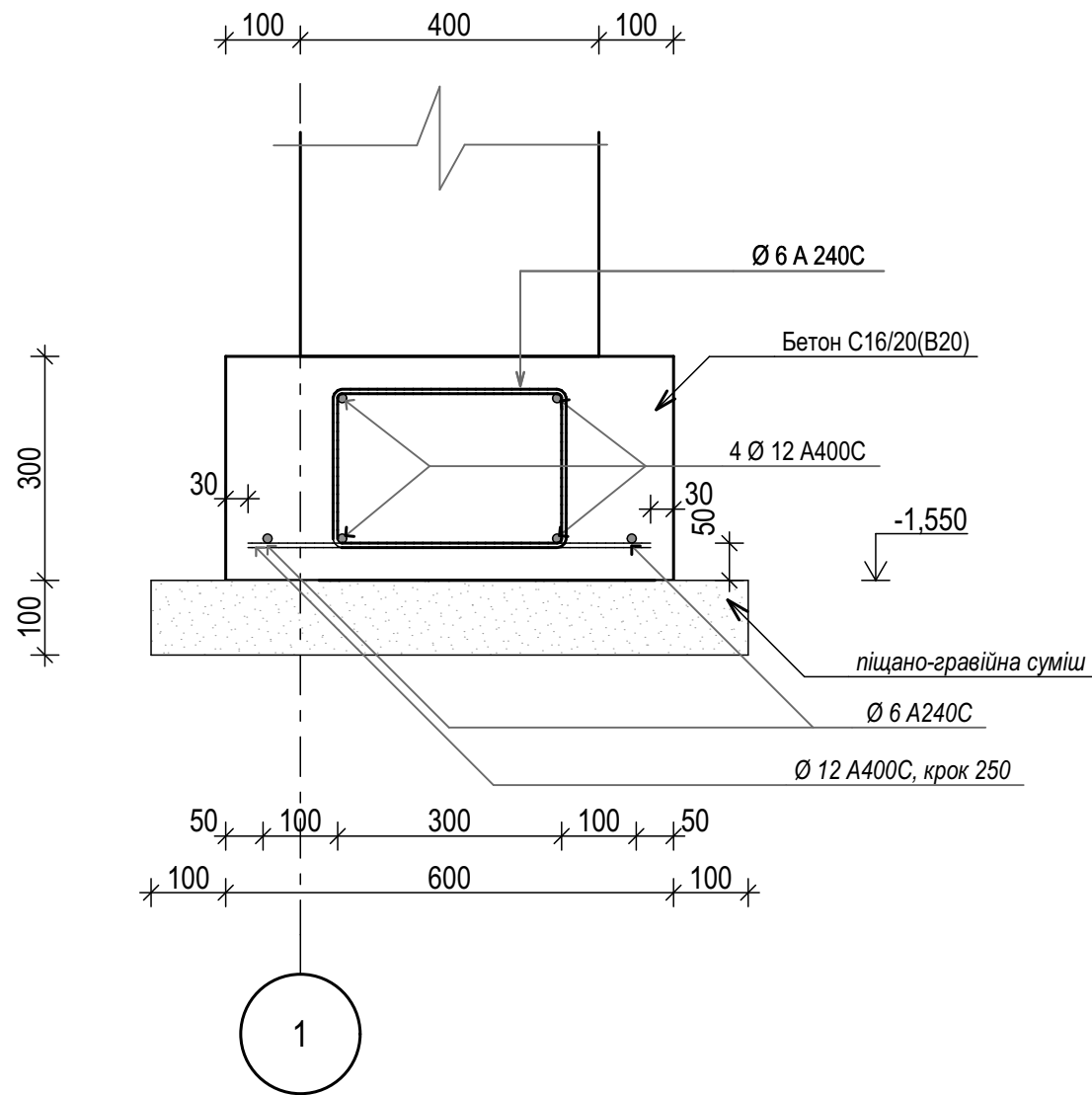
а-а (Деталь 1)
