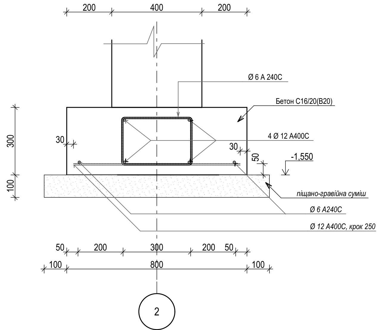
б-б (Деталь 2)
