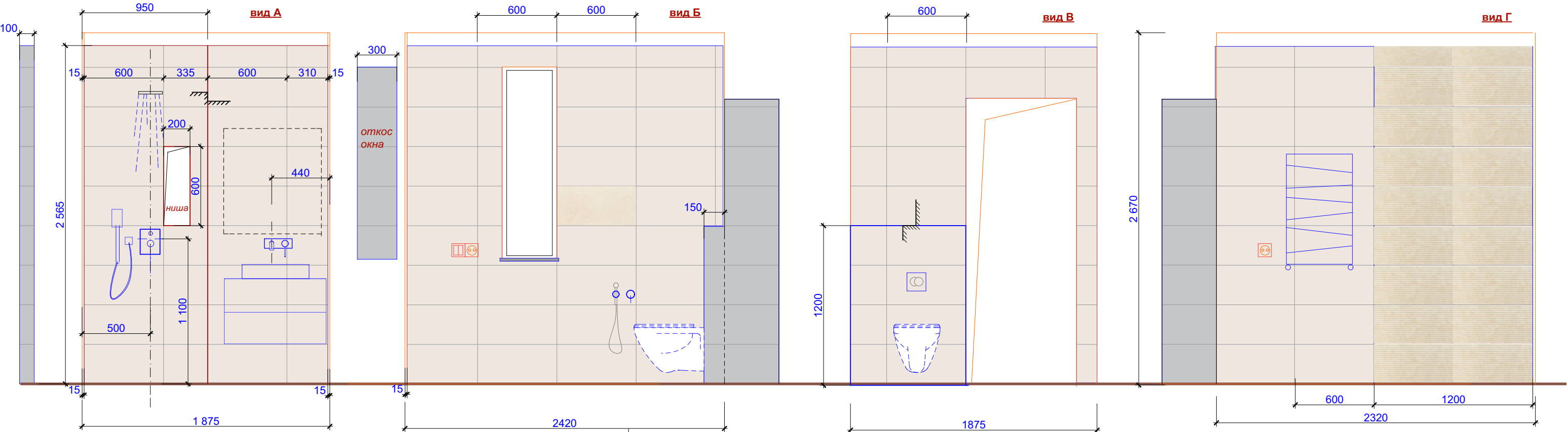
Схема раскладки плитки с/у 2 этажа
