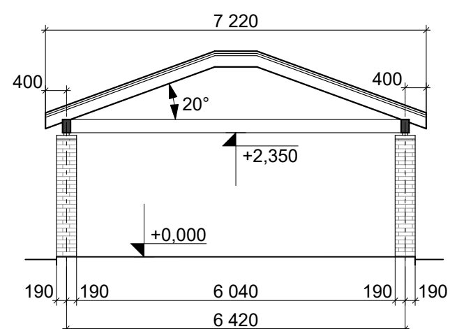
Розріз Б-Б
