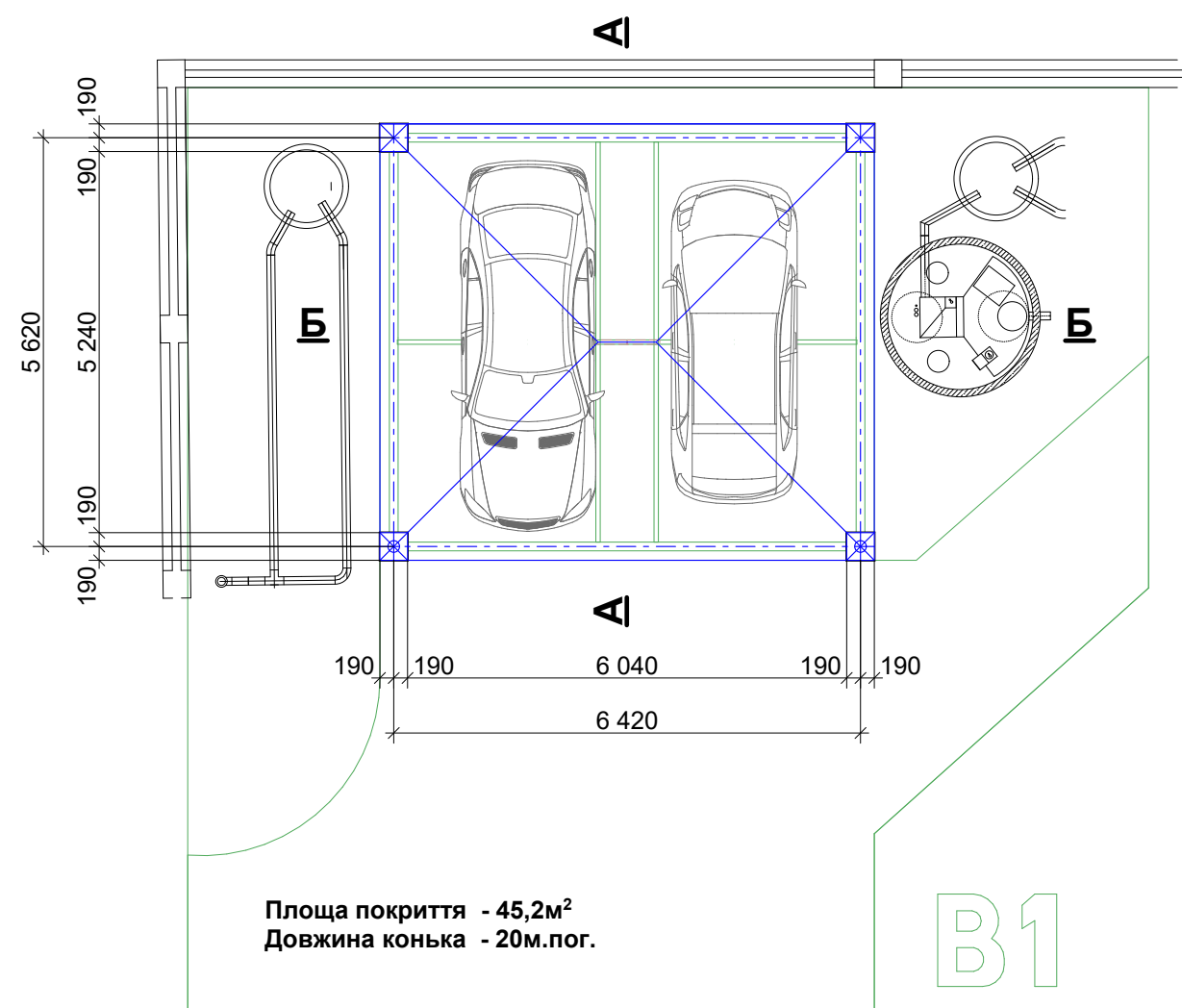
План навісу Вар.1
