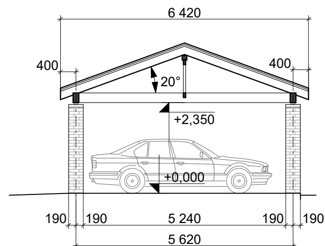
Розріз А-А
