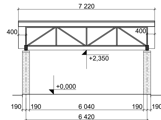
Розріз В-В
