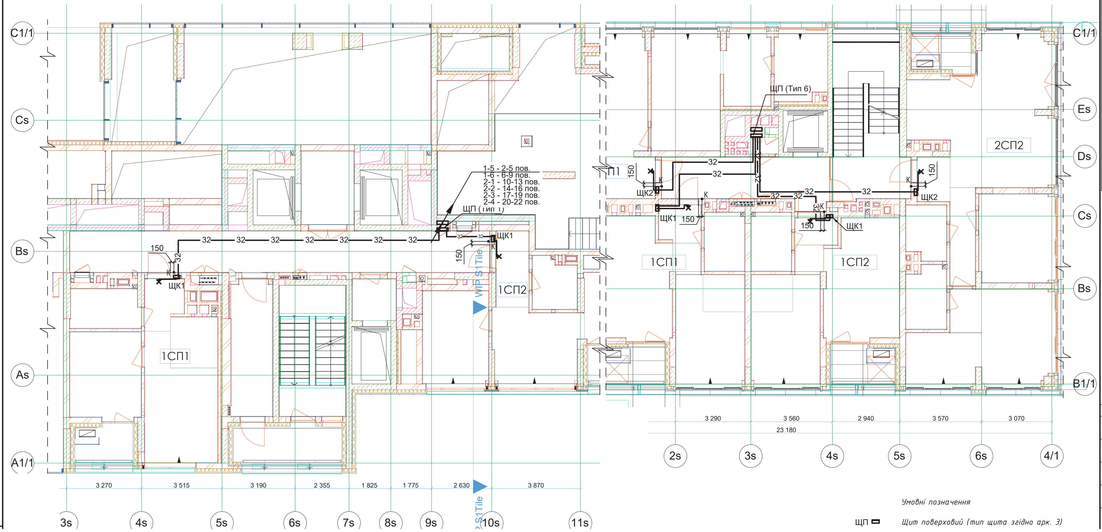
Секція 01 План 2-го поверху
