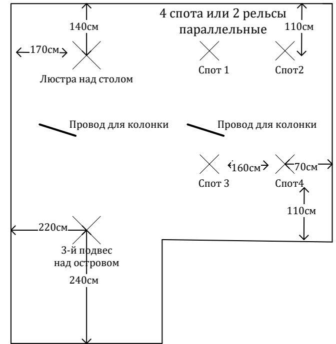
Гостиная
