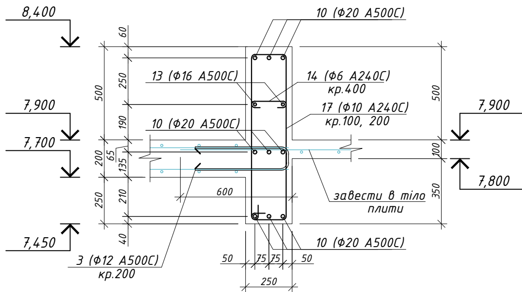
11.1-11.1 (армування)
