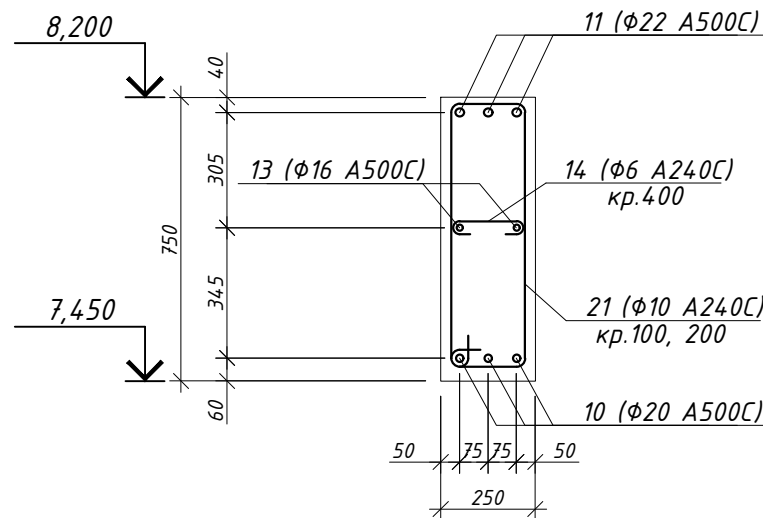
6-6 (армування)
