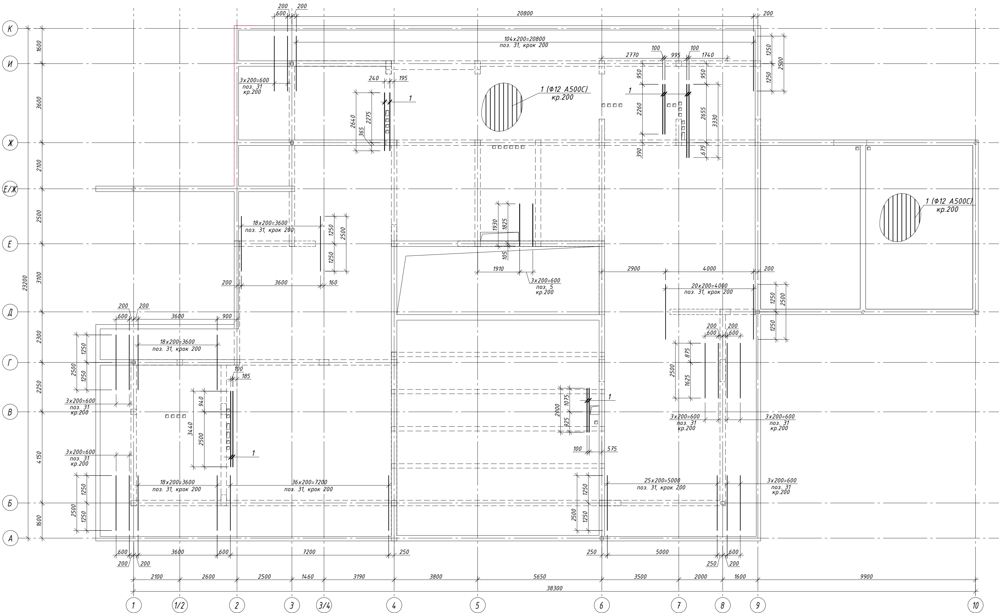
Схема розташування верхньої арматури вздовж цифрових осей плити перекрытия 2-го поверху
