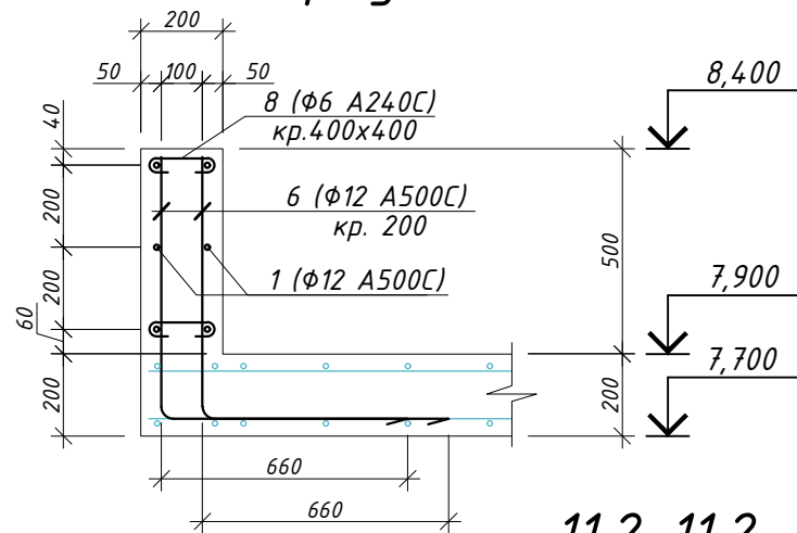
11.2-11.2 (армування)
