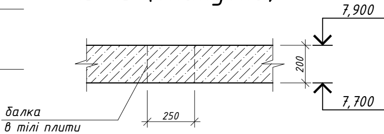
15-15 (опалубка)
