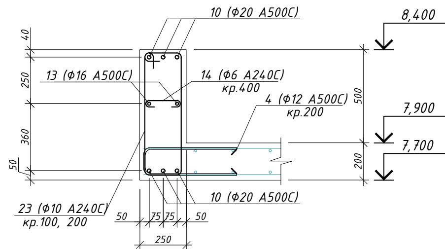
7.2-7.2 (армування)
