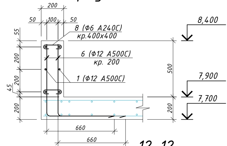
12-12 (армування)
