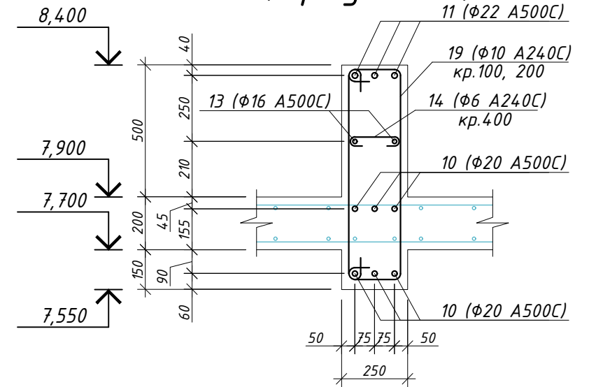
4-4 (армування)
