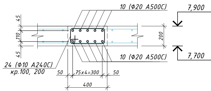
11.1-11.1 (армування)
