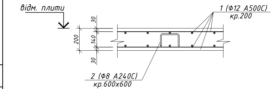
2.1-2.1 (армування)
