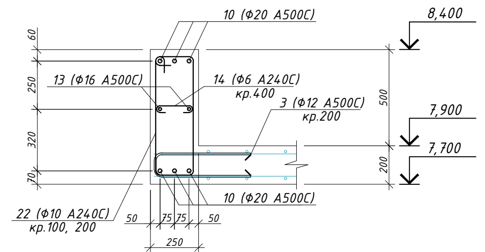
7.1-7.1 (армування)
