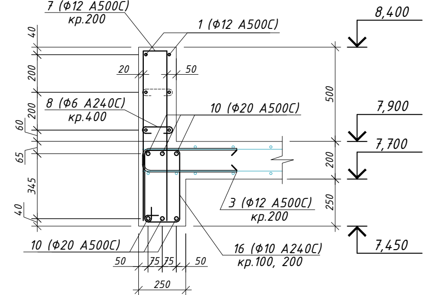
12-12 (армування)
