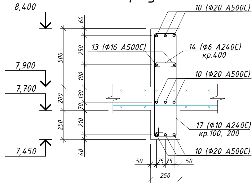
5-5 (армування)
