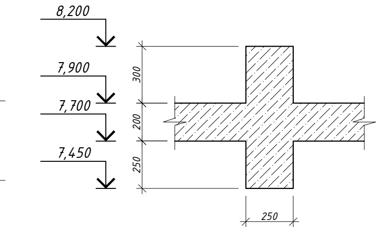
13-13 (опалубка)
