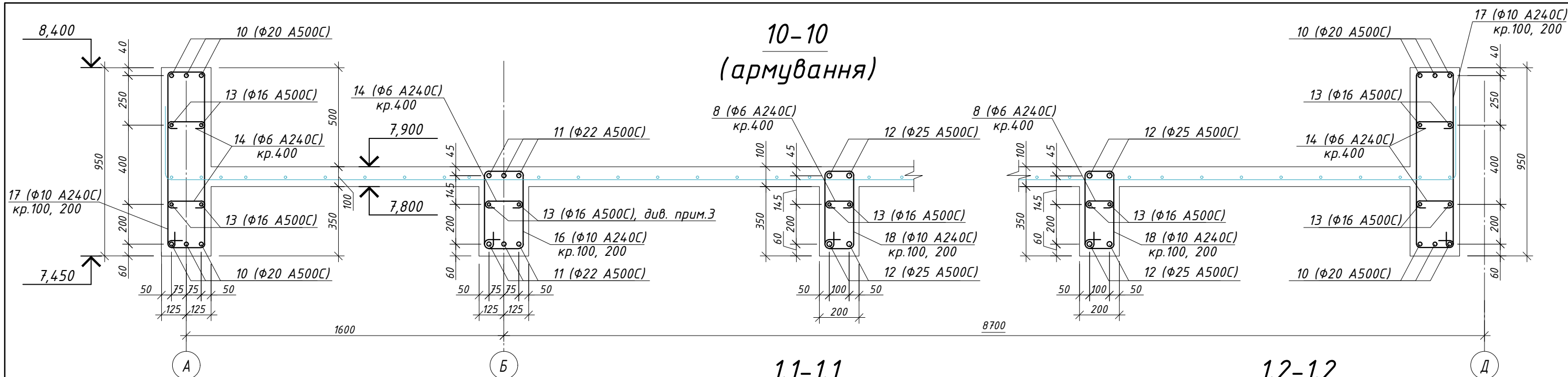
Вузол фіксації верхньої арматури
