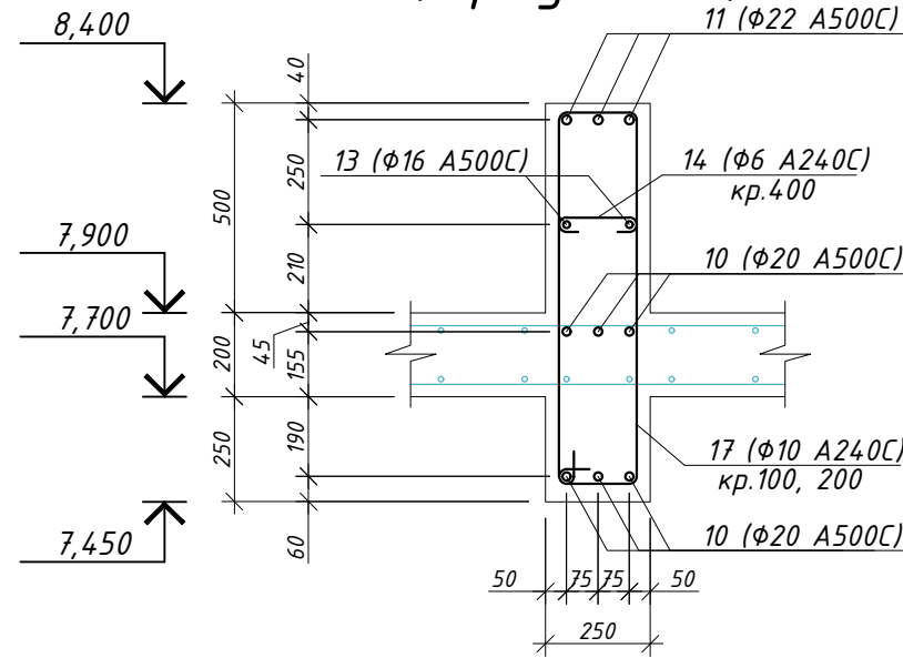
3.2-3.2 (армування)
