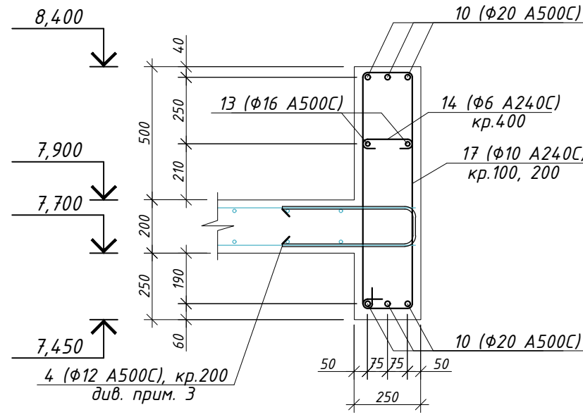
11.2-11.2 (армування)
