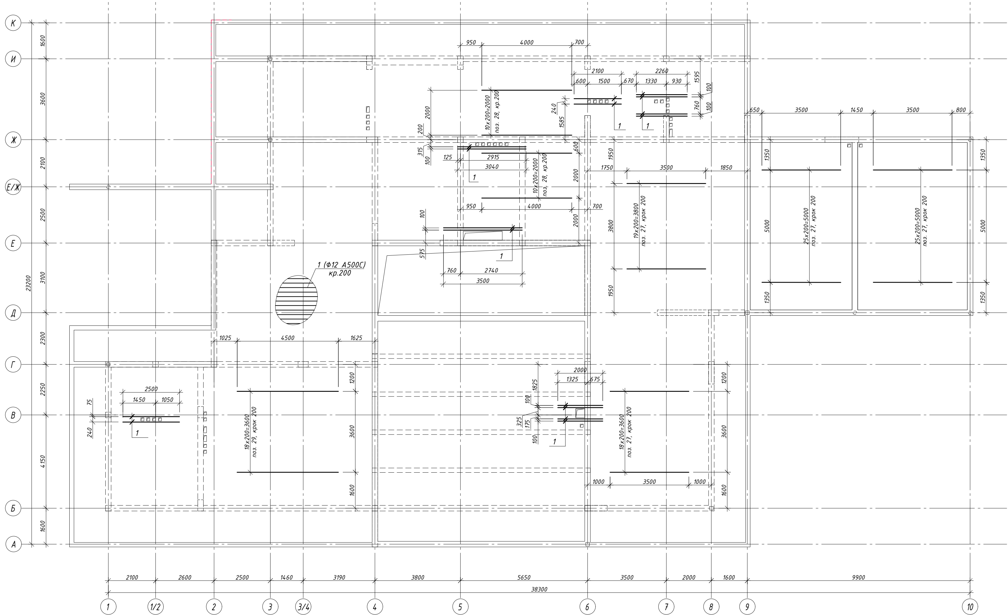
Схема розташування нижньої арматури вздовж літерних осей плити перекрытия 2-го поверху
