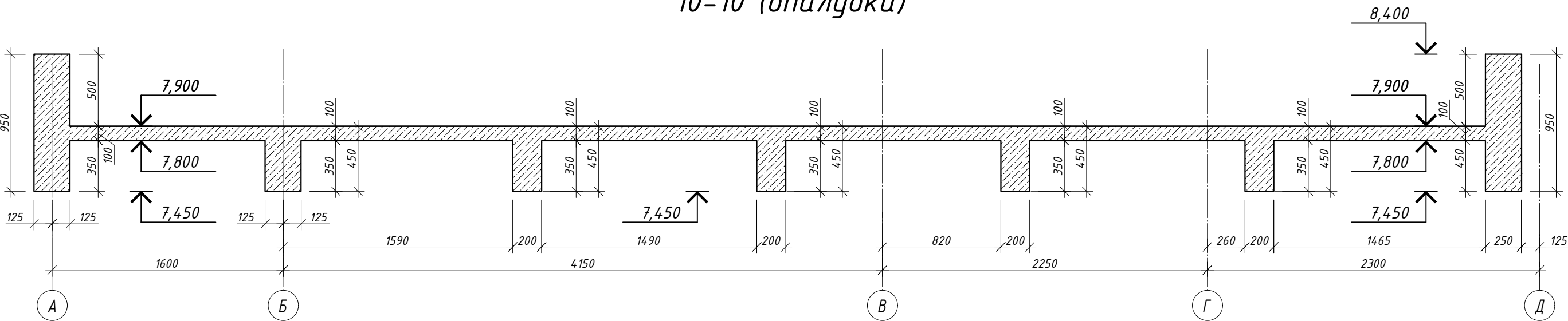
10-10 (опалубка)
