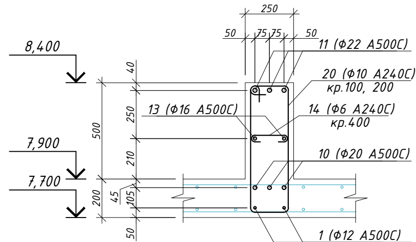
5-5 (армування)
