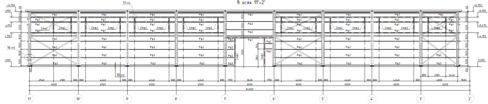
Схема розташування елементів факхверку в осях 11'-2'
