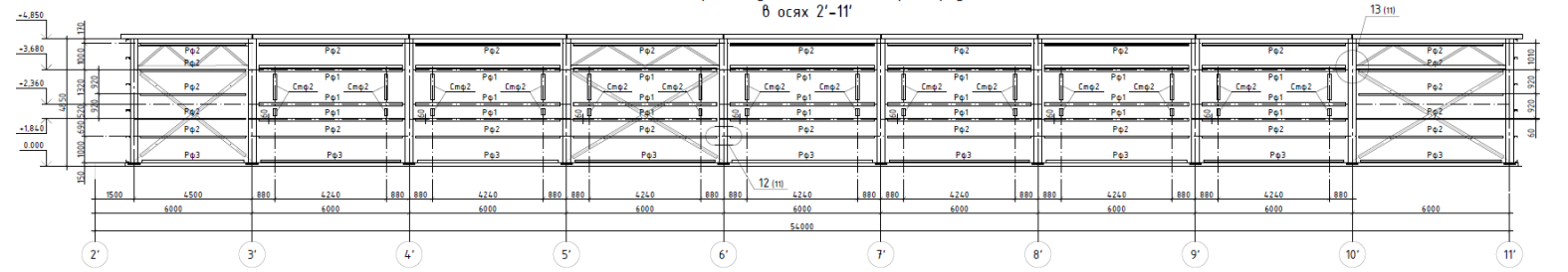
Схема розташування елементів факхверку в осях 11'-2'
