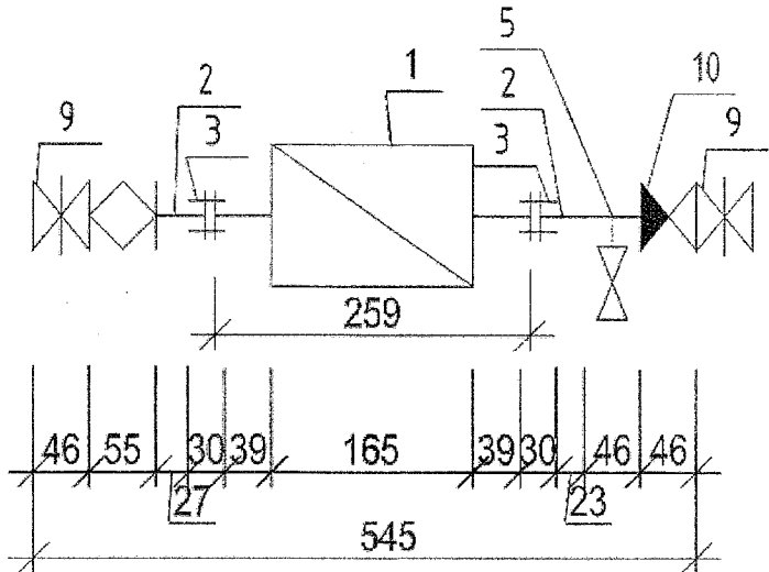
Водомірний вузол ВУ-3 (для офісної частини, поливу), з лічильником холодної води DN = 15 (G = 1/2 ")
