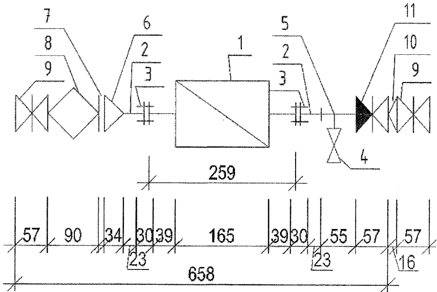
Водомірний вузол ВУ-2 (для житлової частини), з лічильником холодної води DN = 15 (G = 1/2 ")
